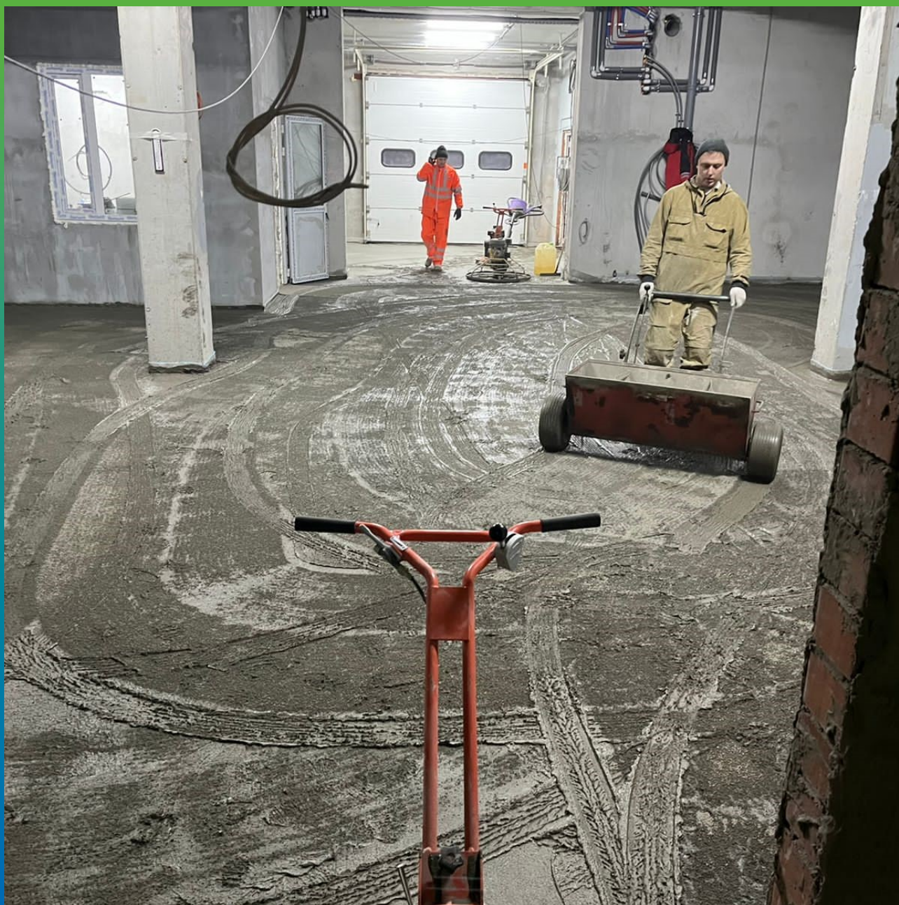
Нанесение Стармекс Топ КР посредством скридбокса
