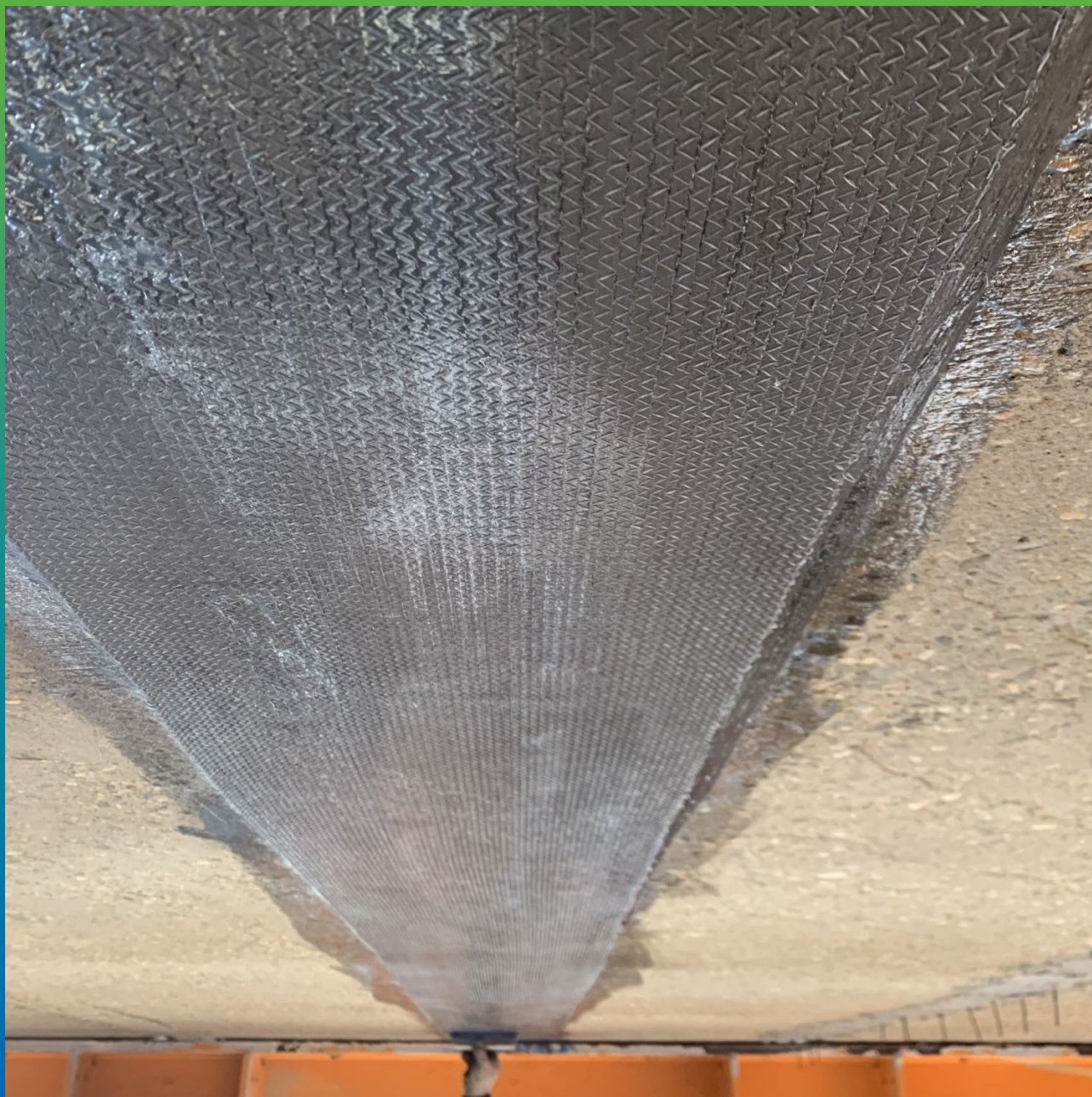
Вид смонтированного углеродного холста Армошел KB200 на клей Манопокс 183
