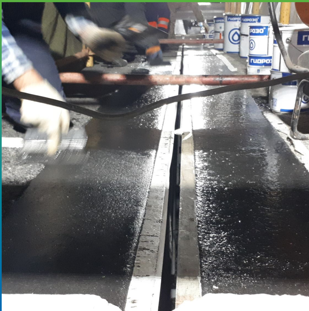
Заполнение шва полиуретановым составом Манопур 336
