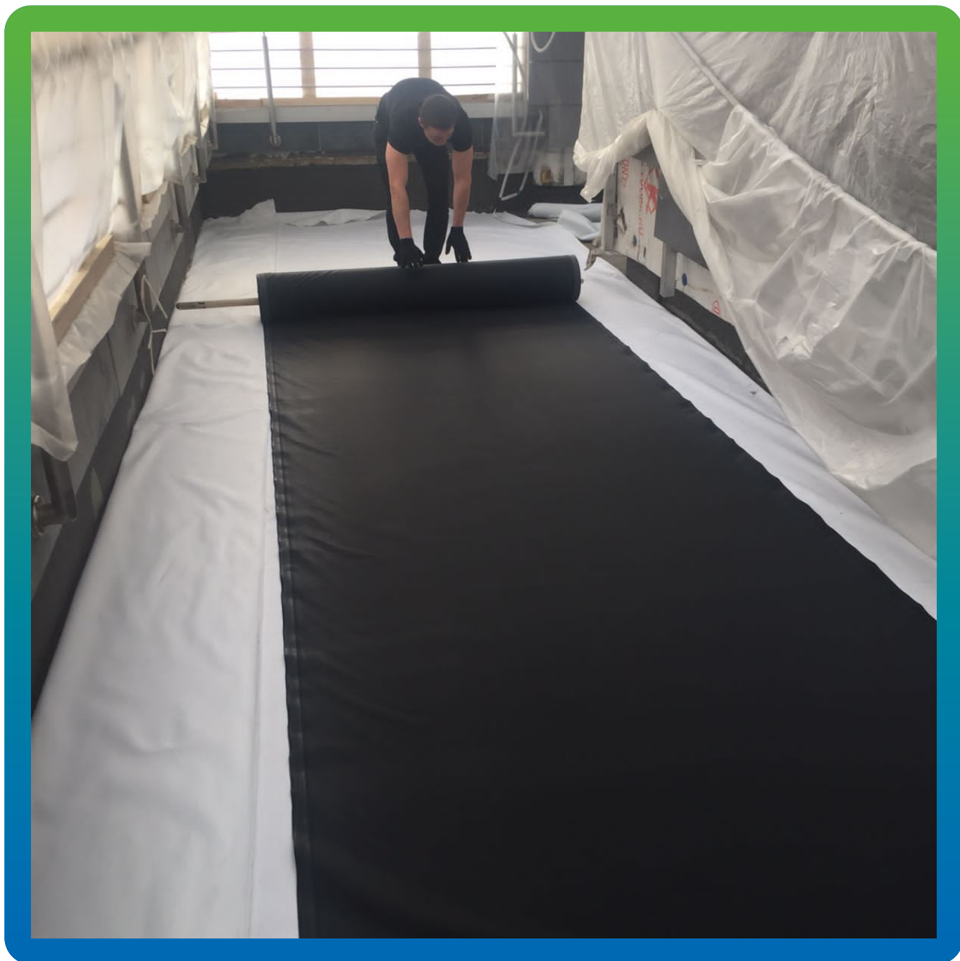
Укладка мембраны Преласты СТ
