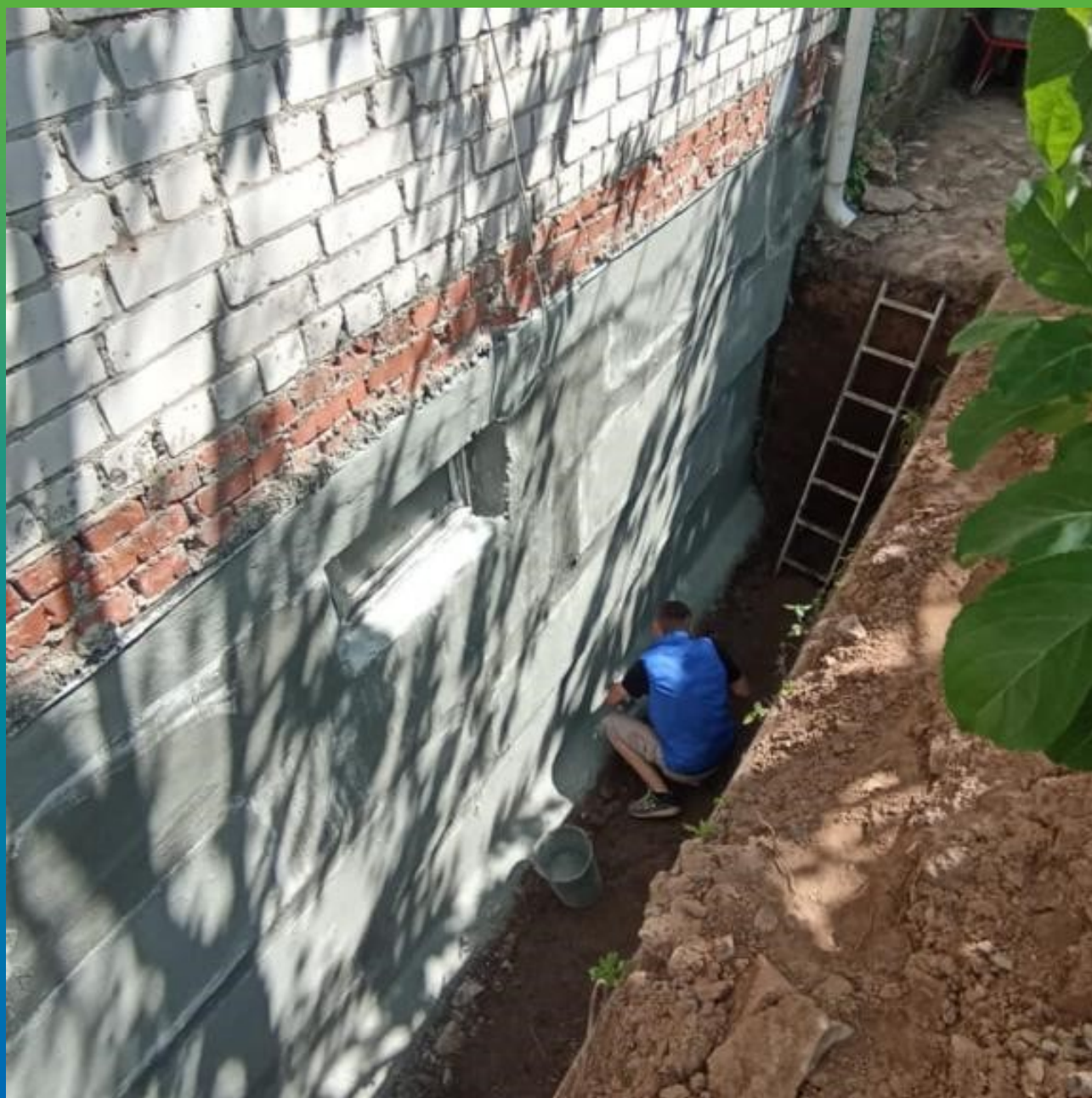
Внешний вид завершеного объекта
