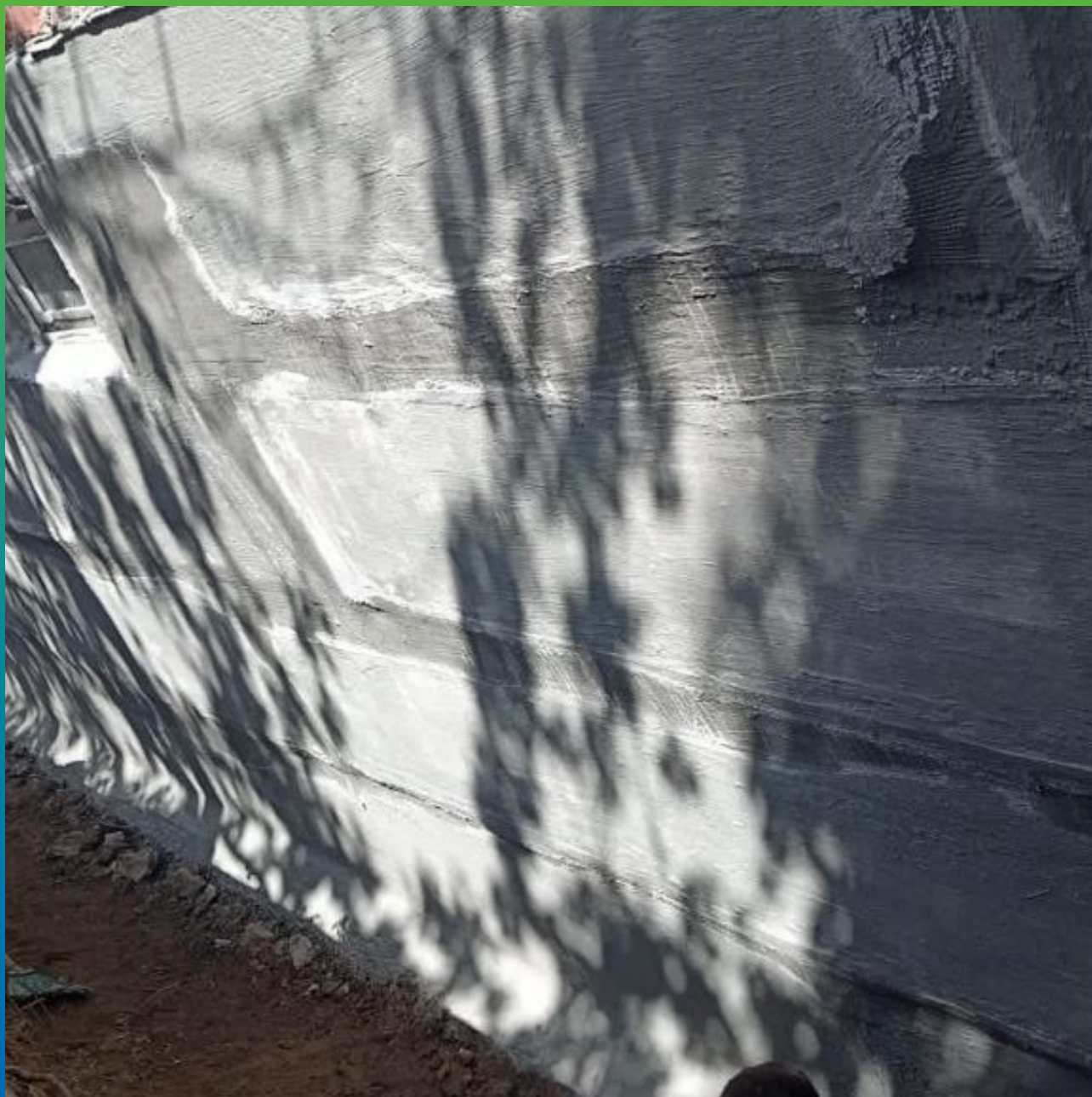
Обмазка швов эластичным составом Стармекс Эласт
