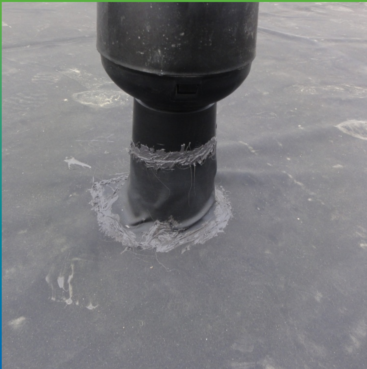
Устройство аэратора
