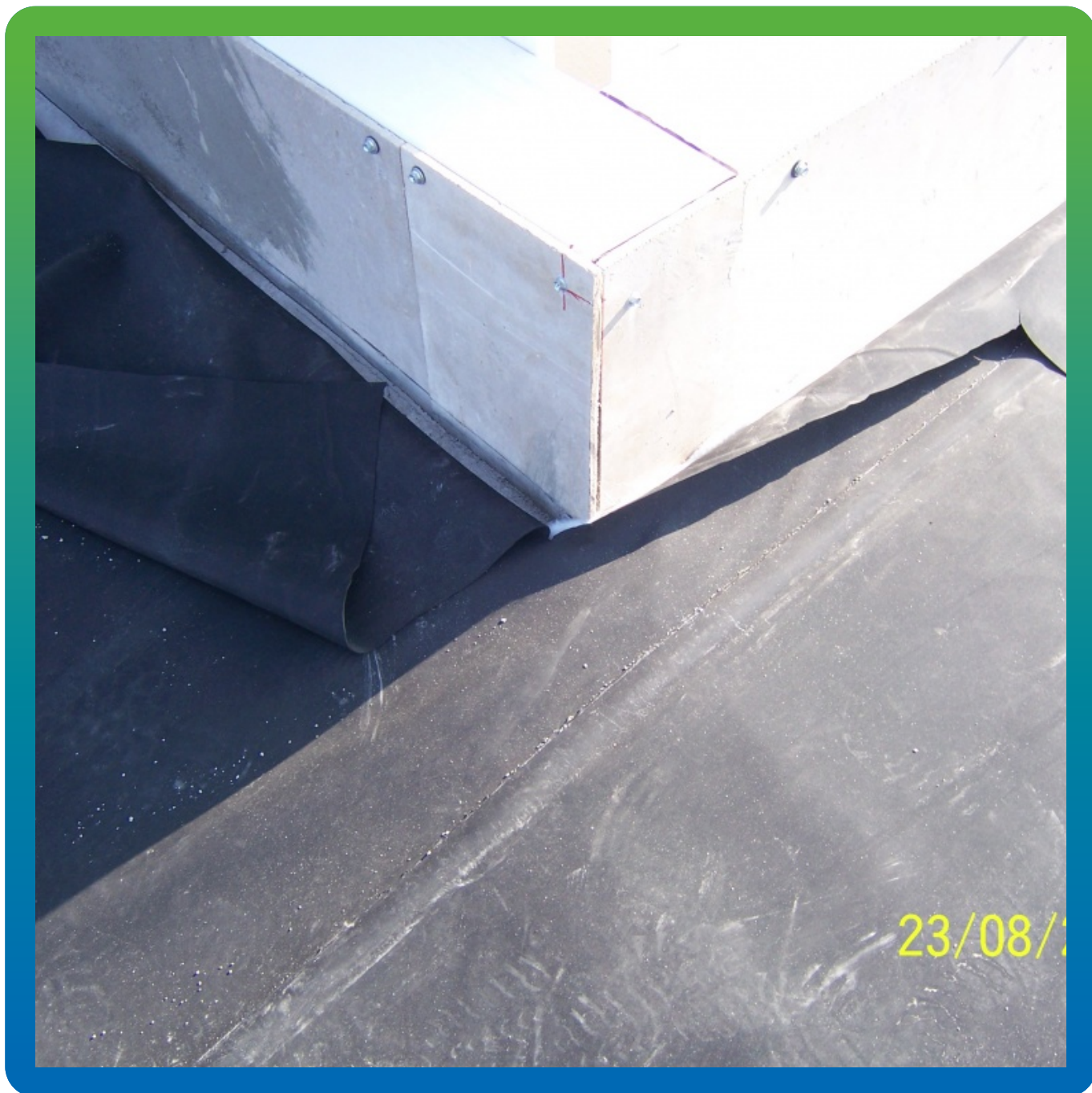
Устройство внешнего угла
