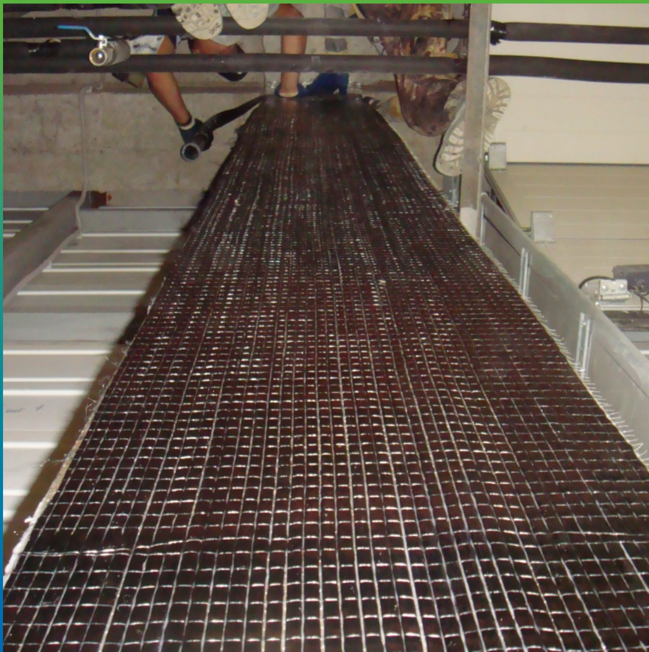
Монтаж поперечных хомутов Тайфо
