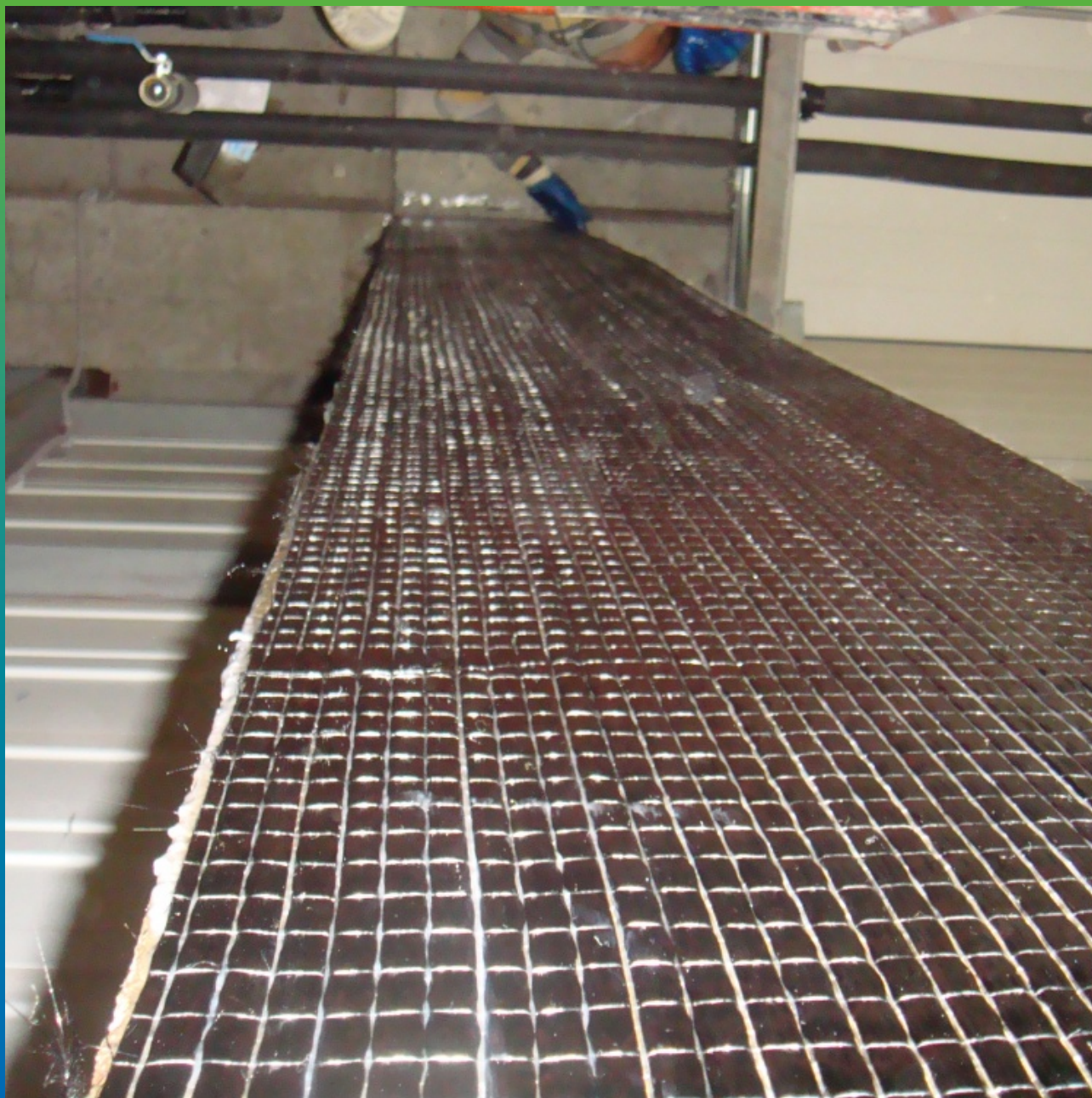
Монтаж холста Тайфо в продольном направлении
