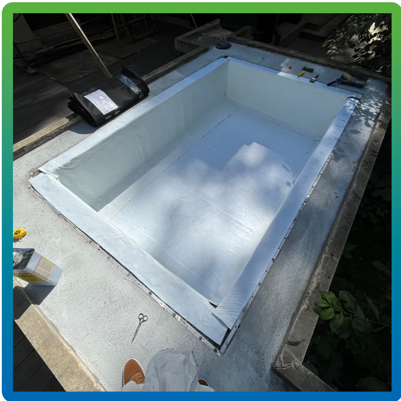
Расстил геотекстиля
