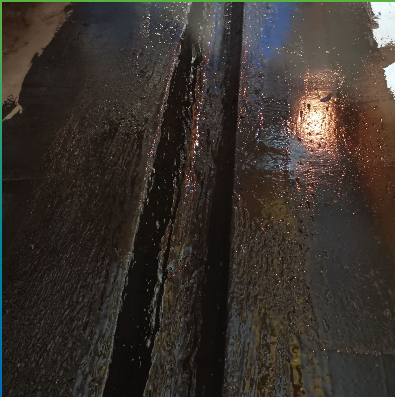
Вид лотка после производства работ по нанесению высокотемпературного покрытия ДенсТоп ПС 391
