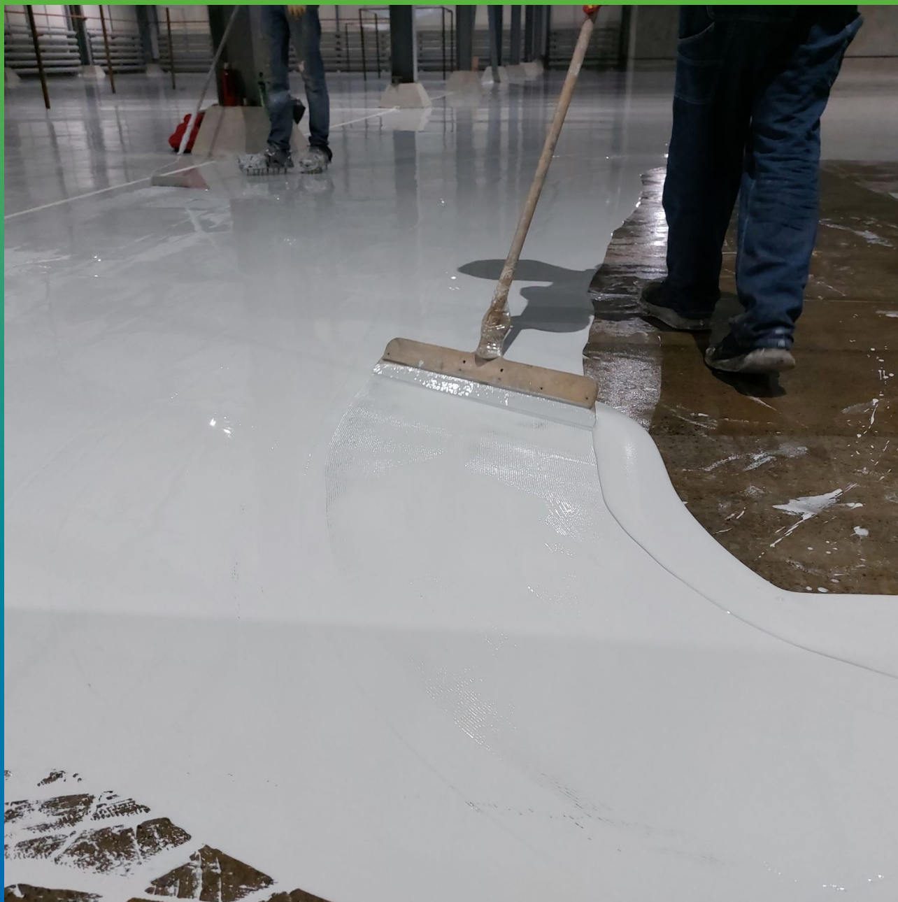
Распределение зубчатым шпателем материала с расходом 1 кг на м 2
