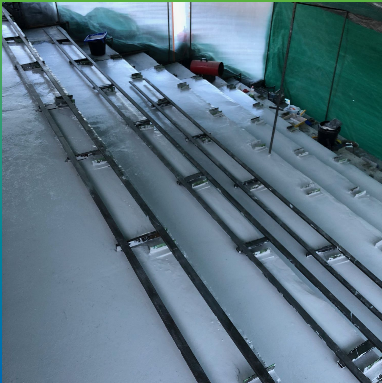
Вид нанесёного защитного покрытия Денстоп ПУ 730 УФ Колор
