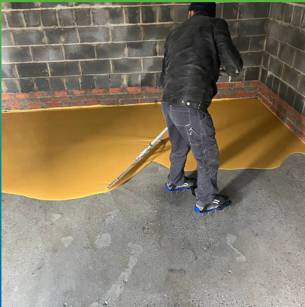
Процесс растягивания материала ракелью с настраиваемой высотой зуба
