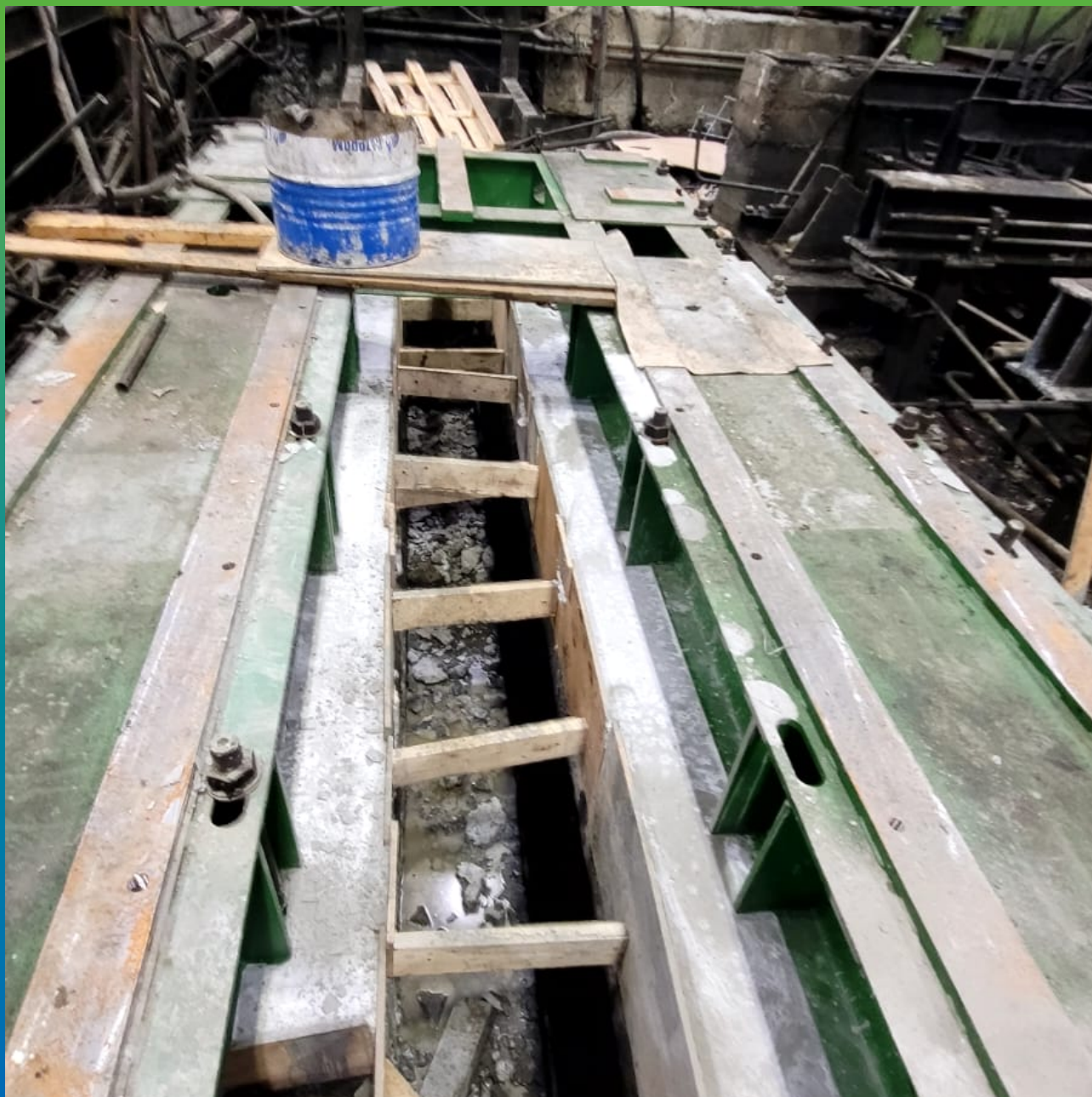
Устройство фундаментного основания под станок составом Стармекс ФМ7
