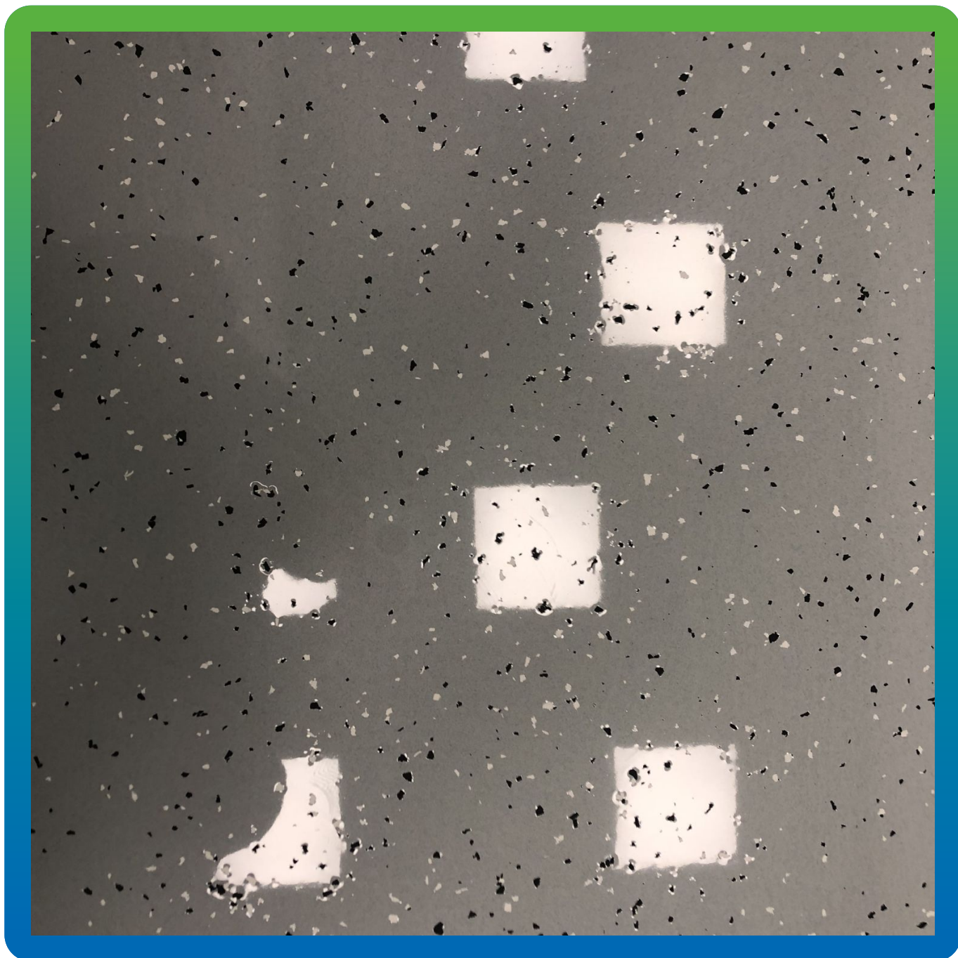
Уложенное финишное покрытие ДенТоп ЭП 500 + ДенТоп Флокс СТ
