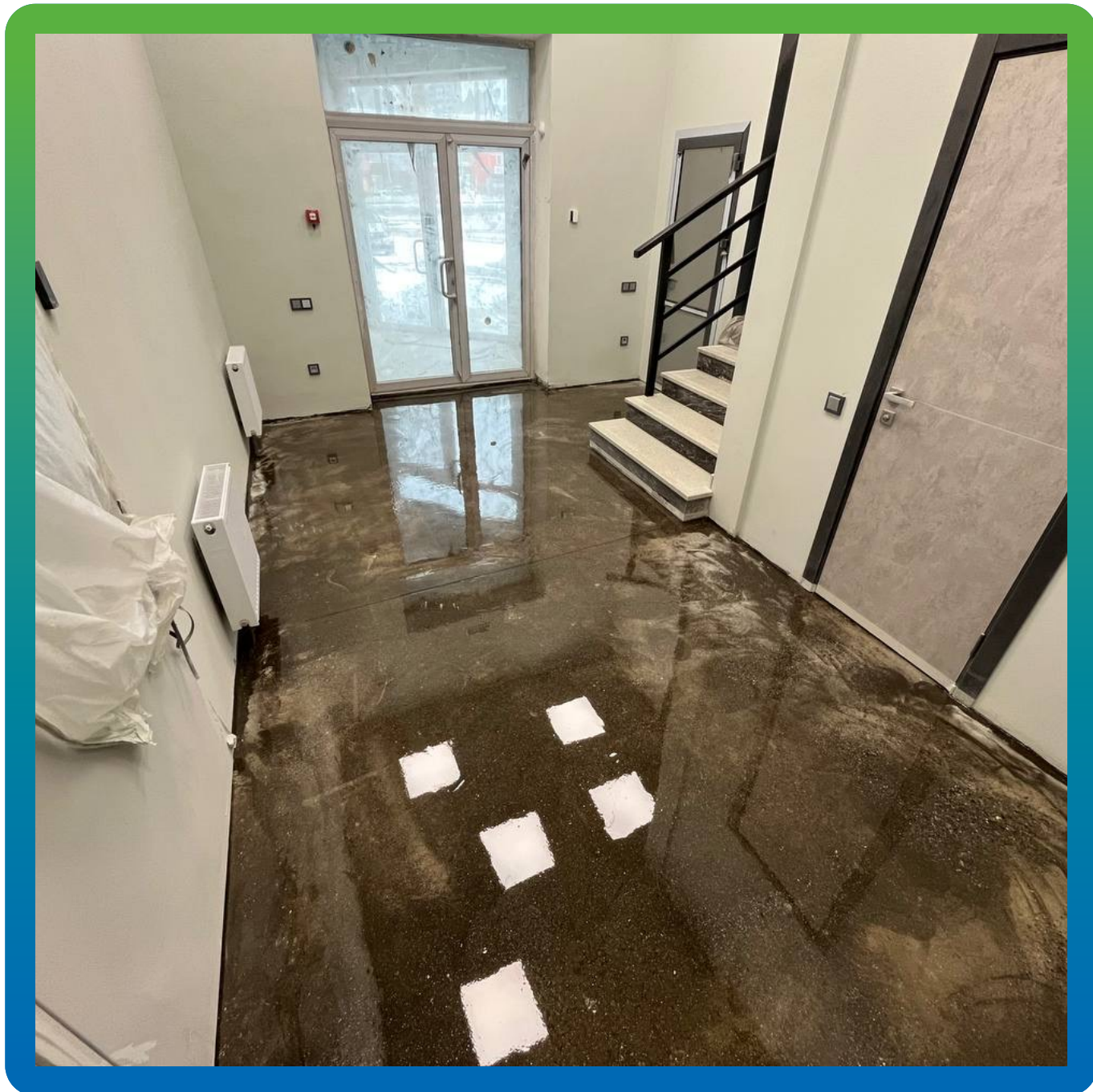
Огрунтованное основания ДенТоп ЭП 106
