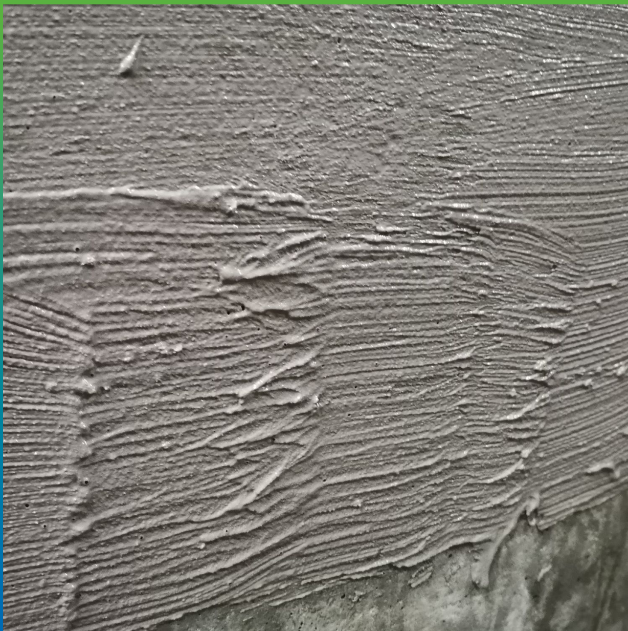
Нанесение второго слоя эластичной гидроизоляции Стармекс Эласт
