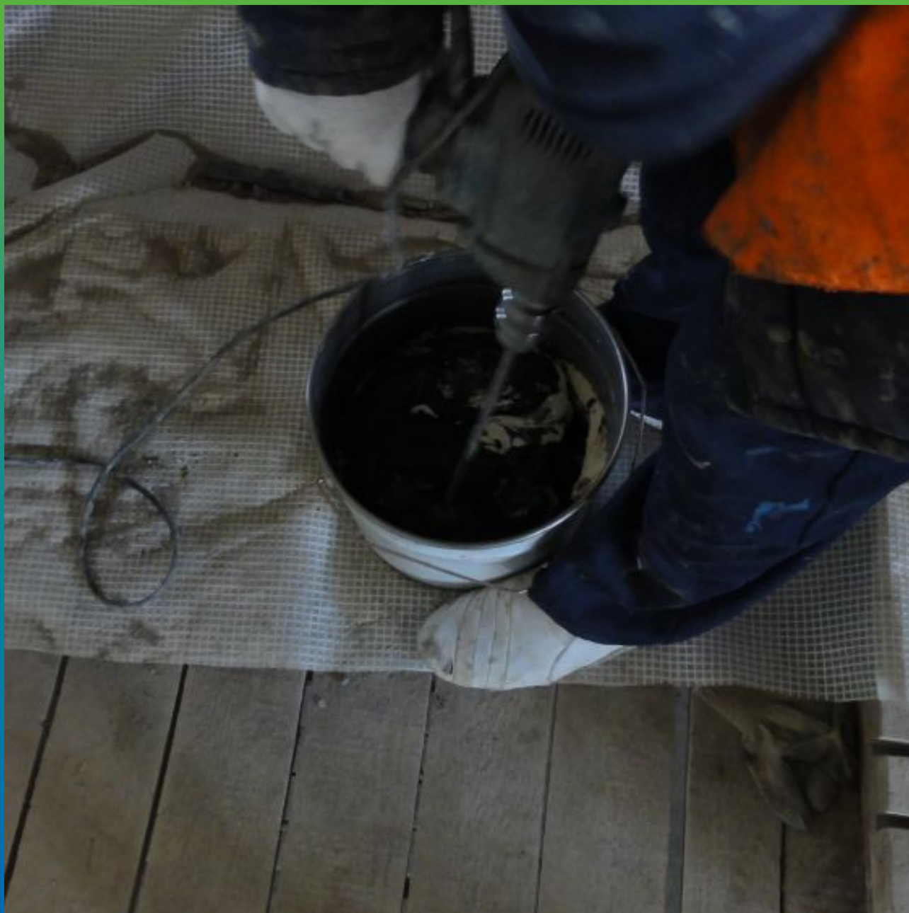
Приготовление ремонтного эпоксидного состава Манопокс 331.
