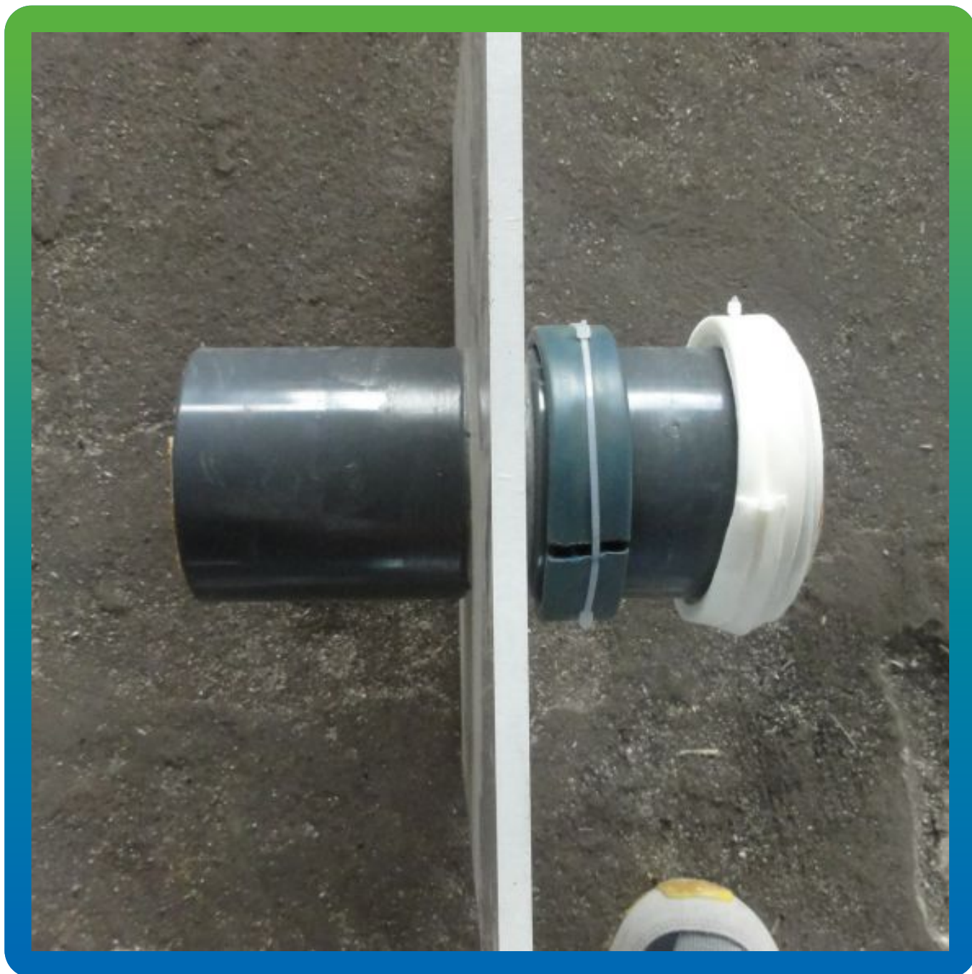
Герметизация ввода коммуникаций профилем Манодил Свелл 2507.
