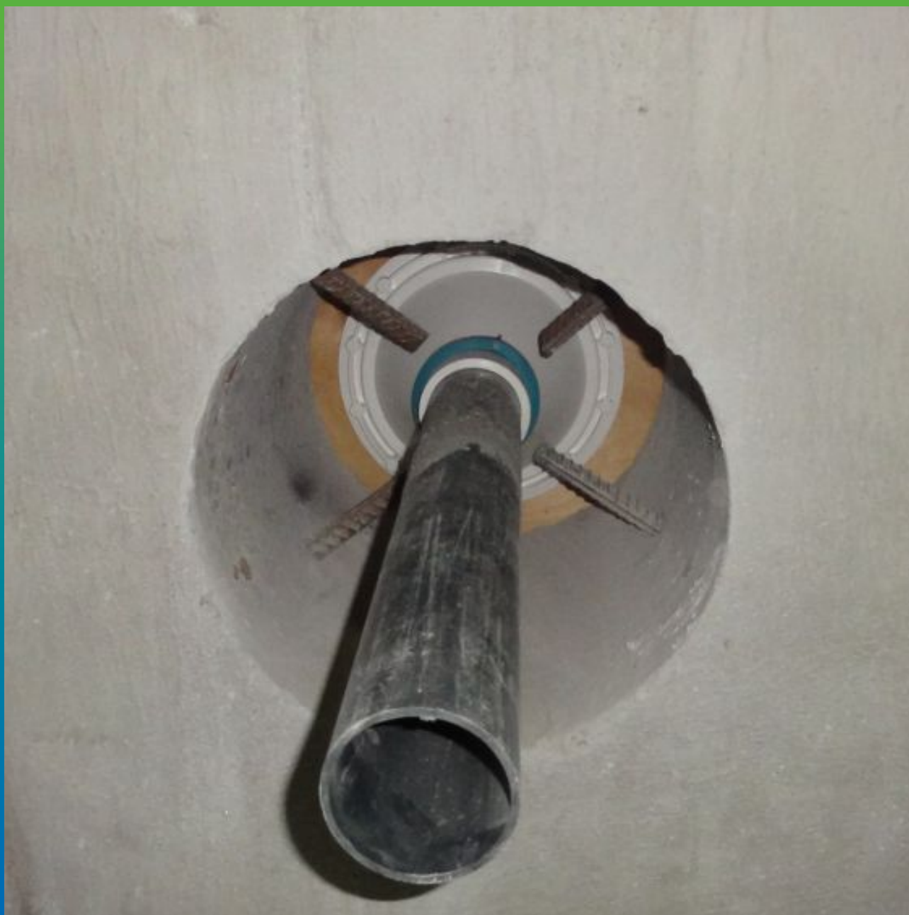
Герметизация ввода коммуникацией профилем Манодил Свелл 2507.
