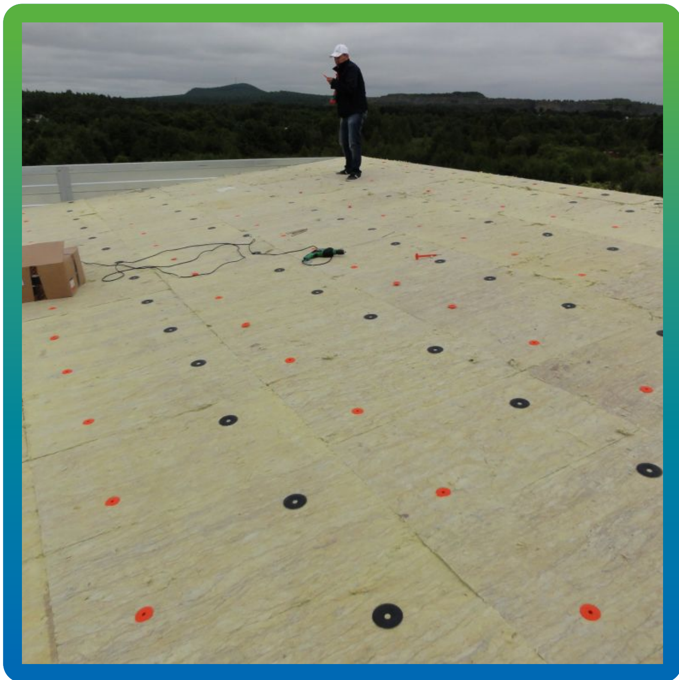
Крепеж утеплителя, установка шайб Центрикс
