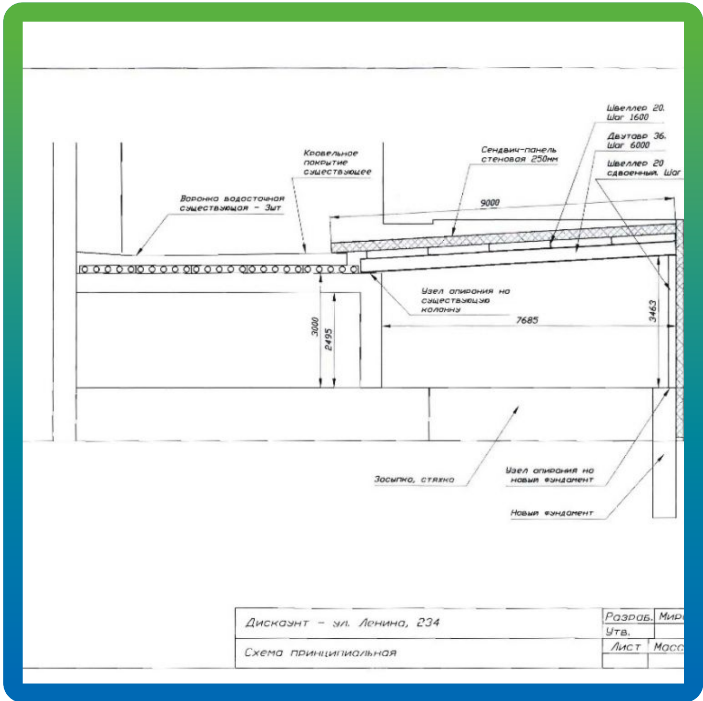
Конструктив кровли
