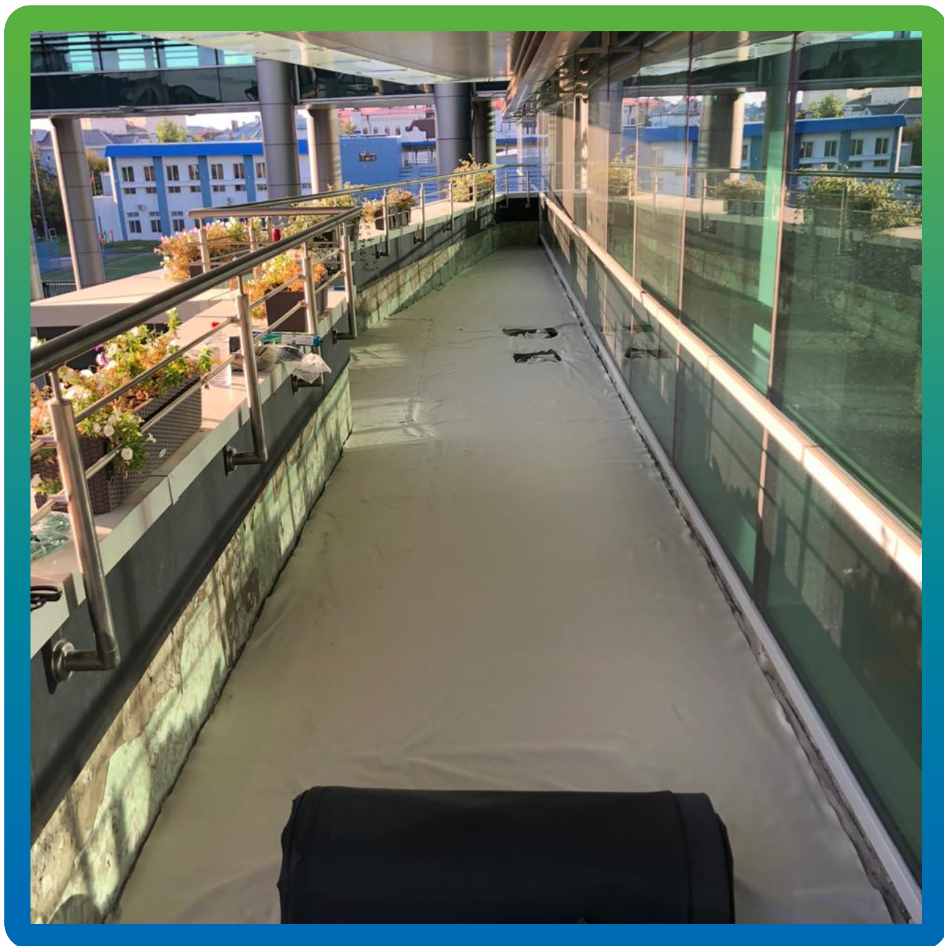
Укладка заранее вулканизированных полотен ЭПДМ мембраны Прелести СТ
