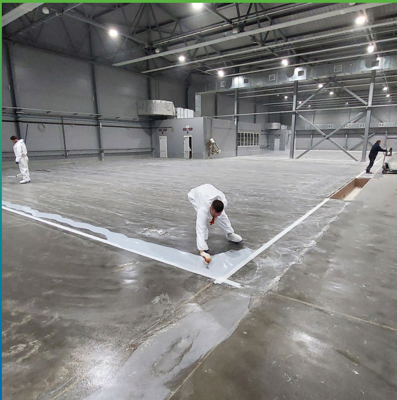
Начало укладки ДенсТоп ЭП 501 на первой захватке
