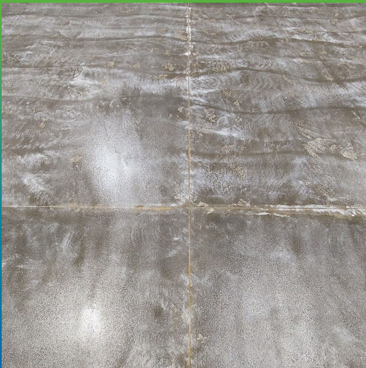
Вид загрунтованной поверхности с последующей подшлифовкой
