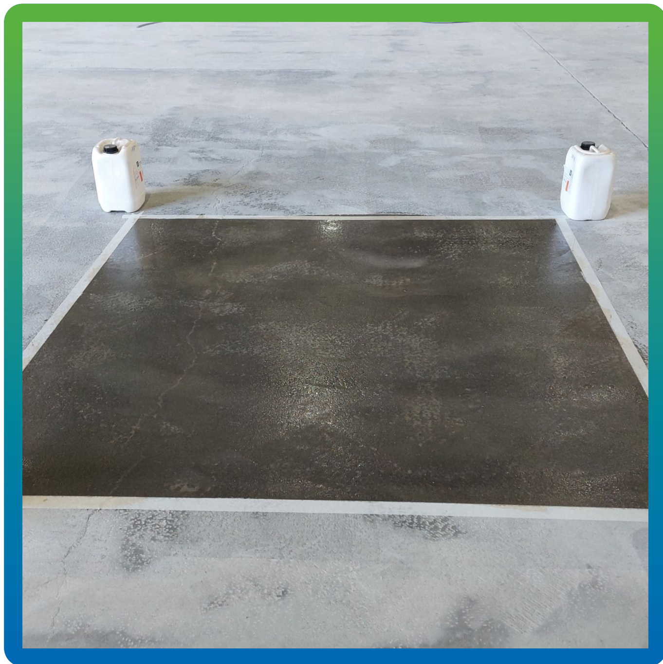
Тестовый участок с грунтовкой ДенсТоп ЭП 100
