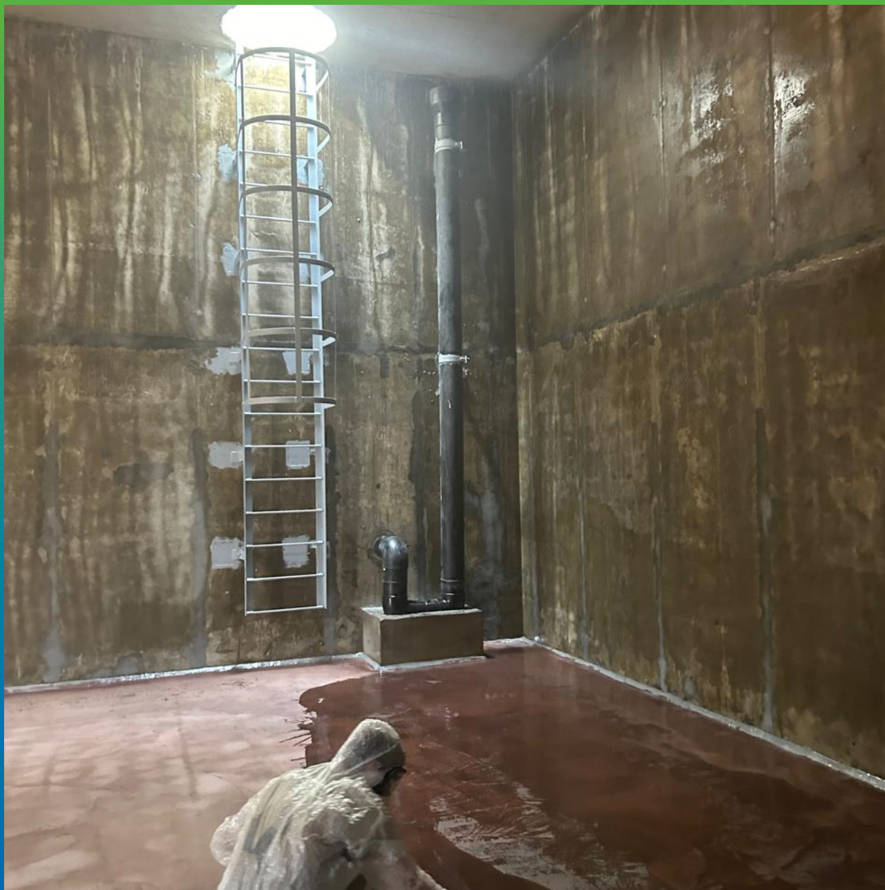
Нанесения грунтовочного слоя ДенсТоп ЭП 100 на пол ручным способом
