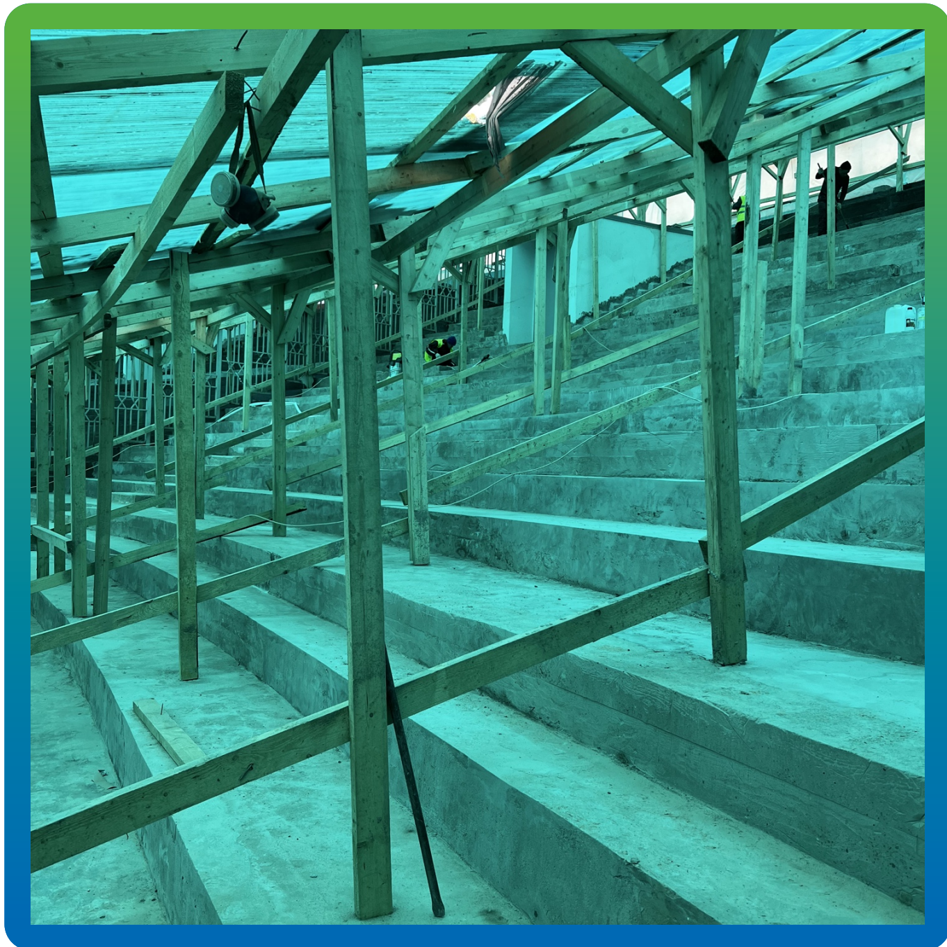
Вид трибун после проведения ремонтных работ и шлифовки
