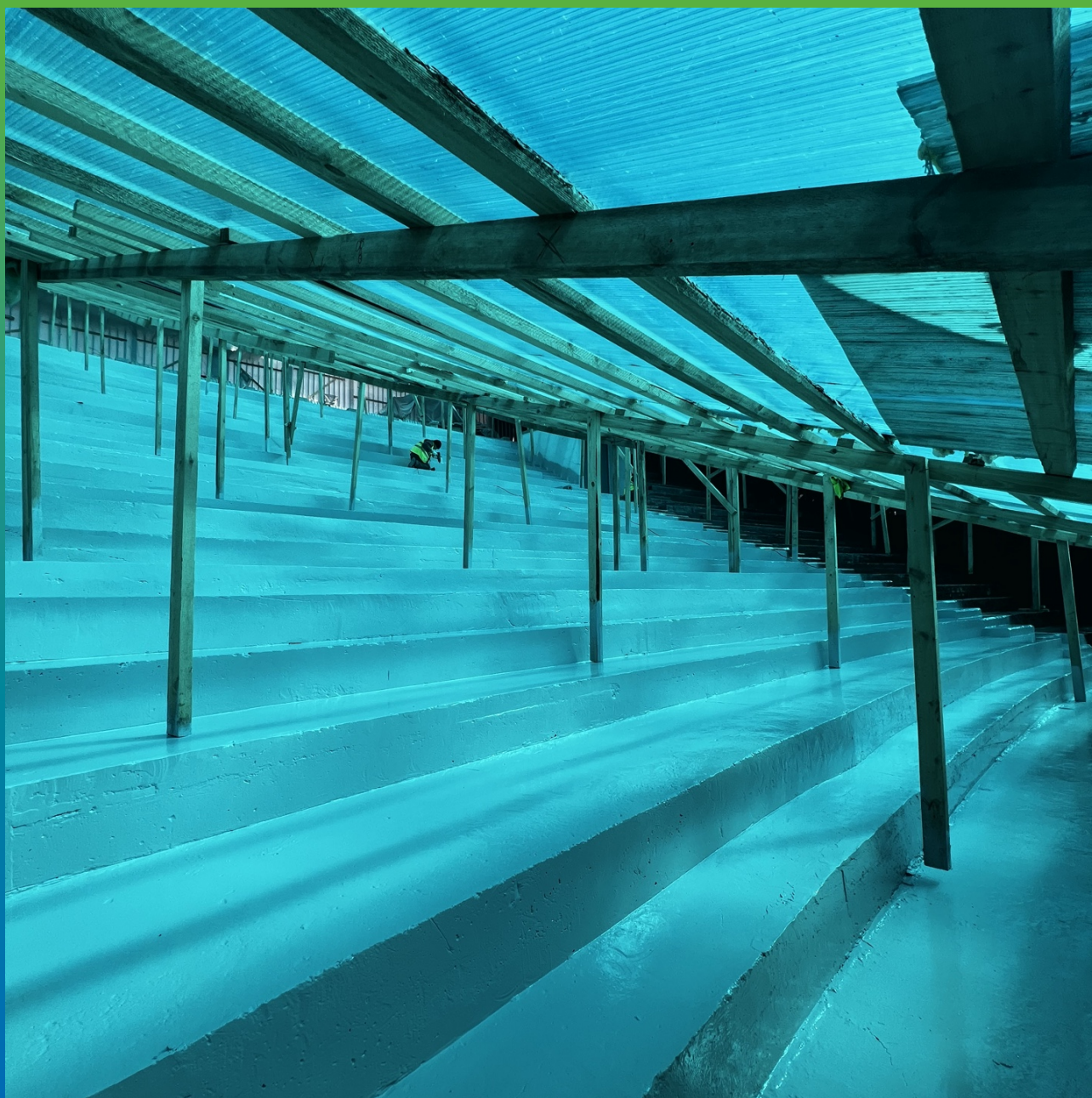
ДенсТоп ПУ 227 Эластик, нанесенный на ж/б трибуны
