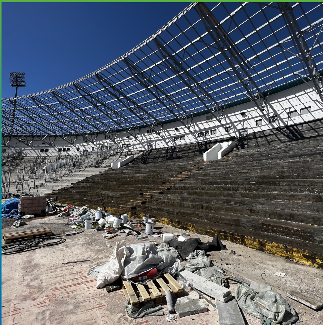
Вид загрунтованной трибуны
