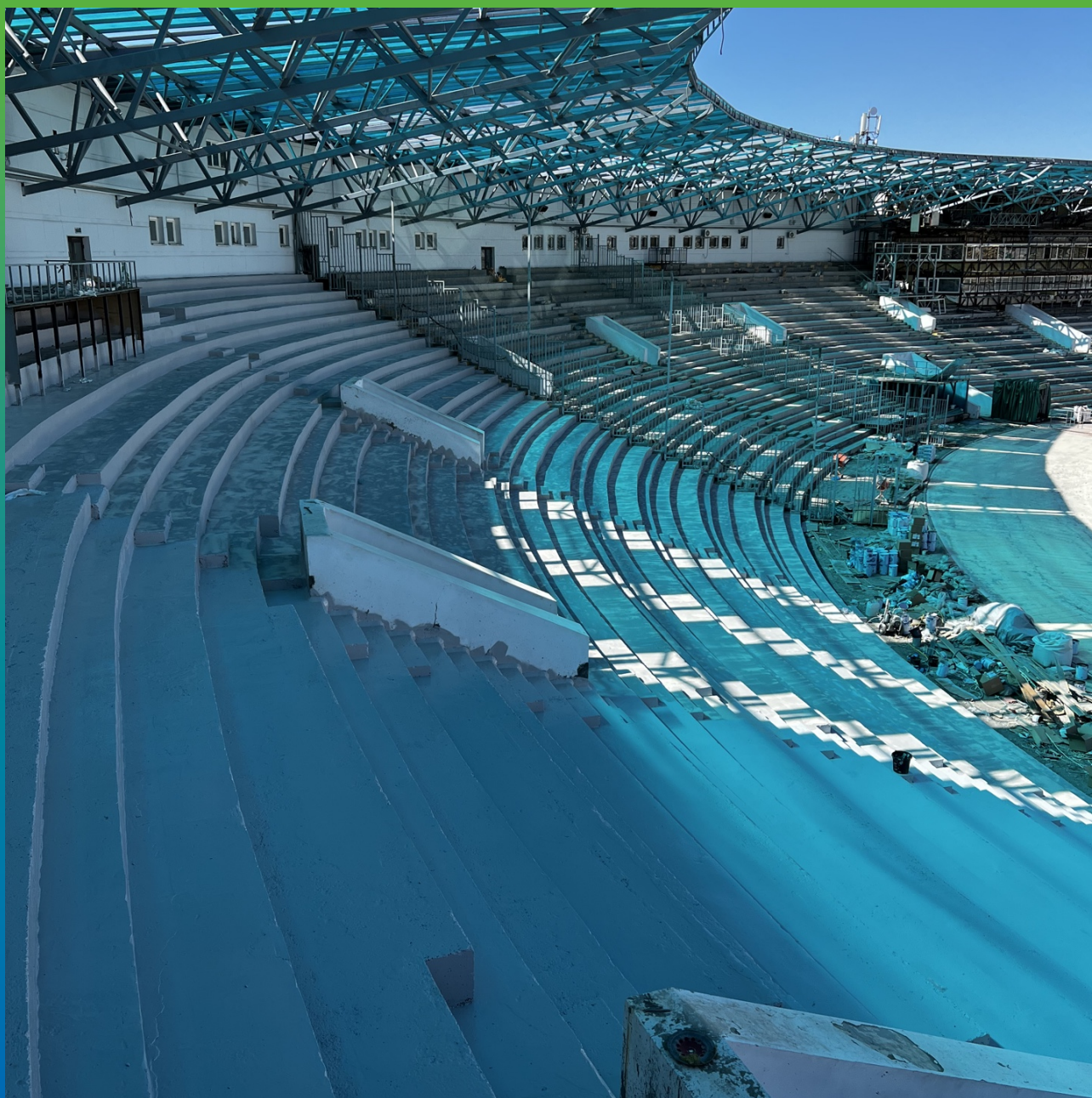
ДенсТоп ПУ 227 Эластик, нанесенный на трибуны
