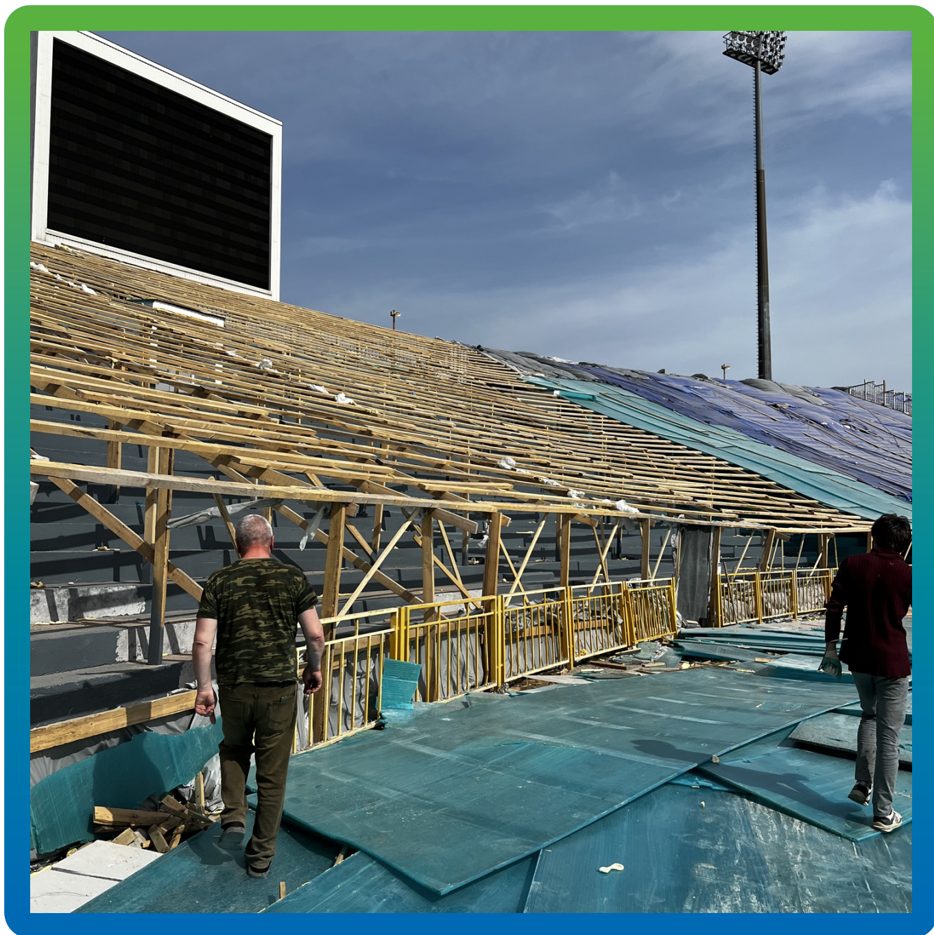
Демонтаж теплового контура
