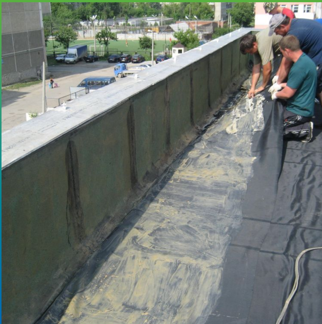
Нанесение адгезива перед приклейкой к парапету
