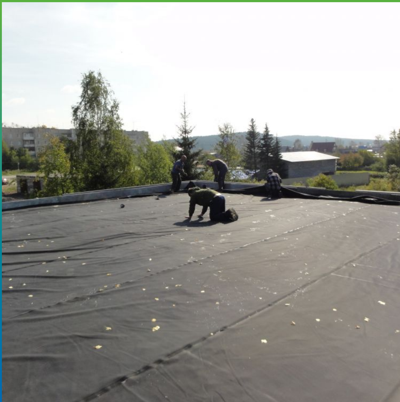
Укладка ЭПДМ Эластосил Т 1.2мм на адгезив П400
