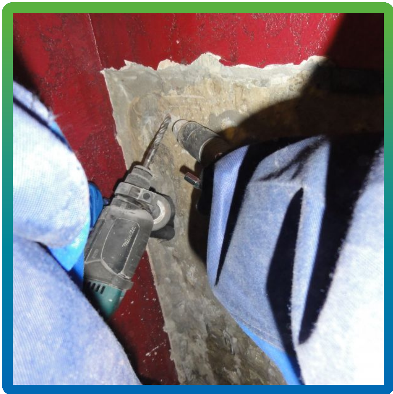
Бурение шпуров под пакера
