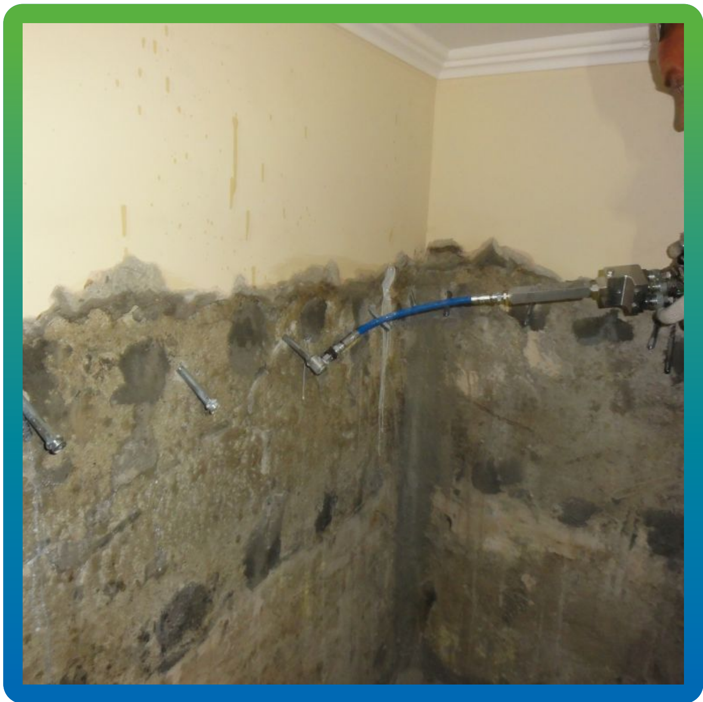
Инъектирование Манокрил Гель В в швы ФБС
