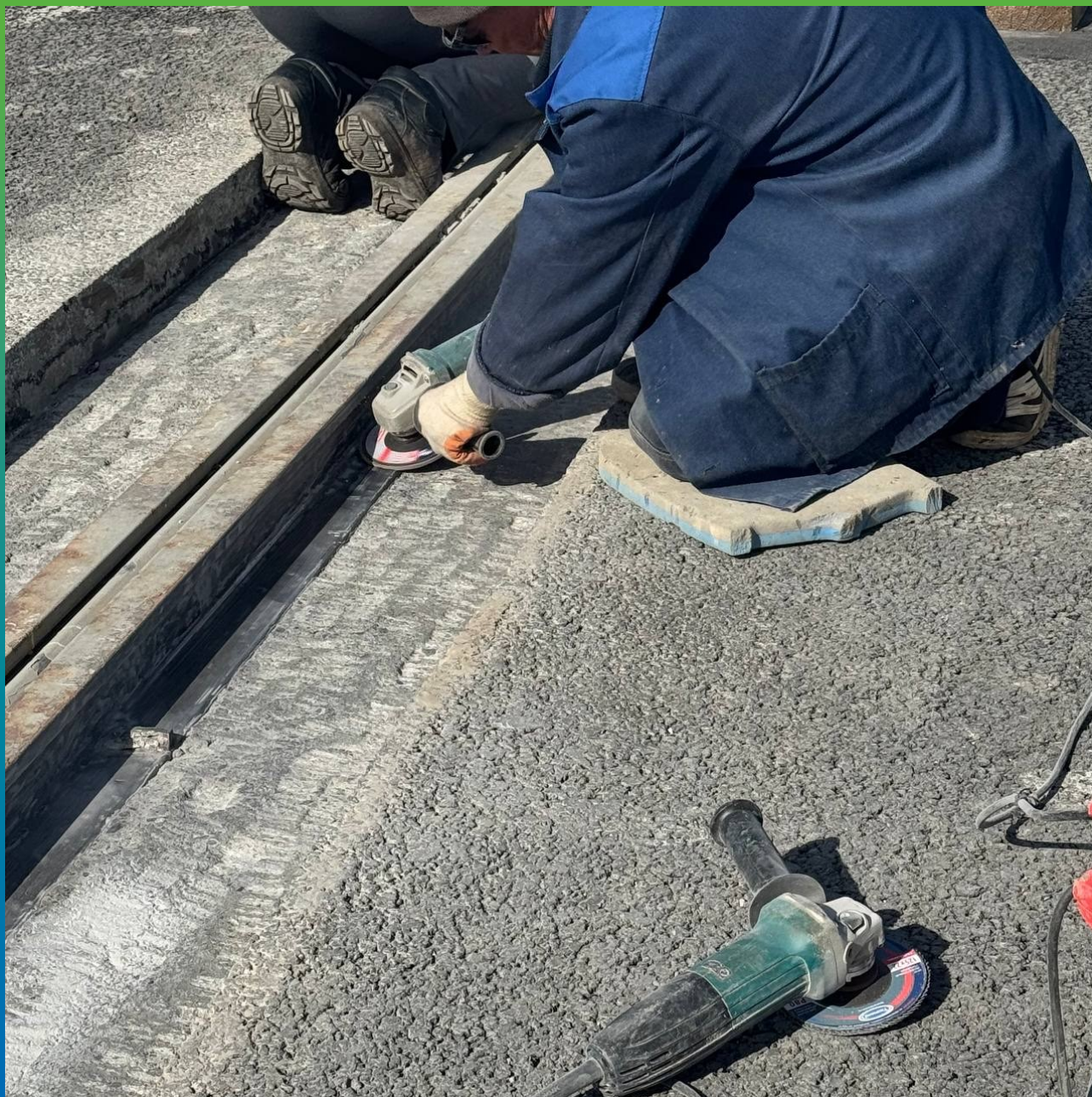
Очистка металлического профиля шва
