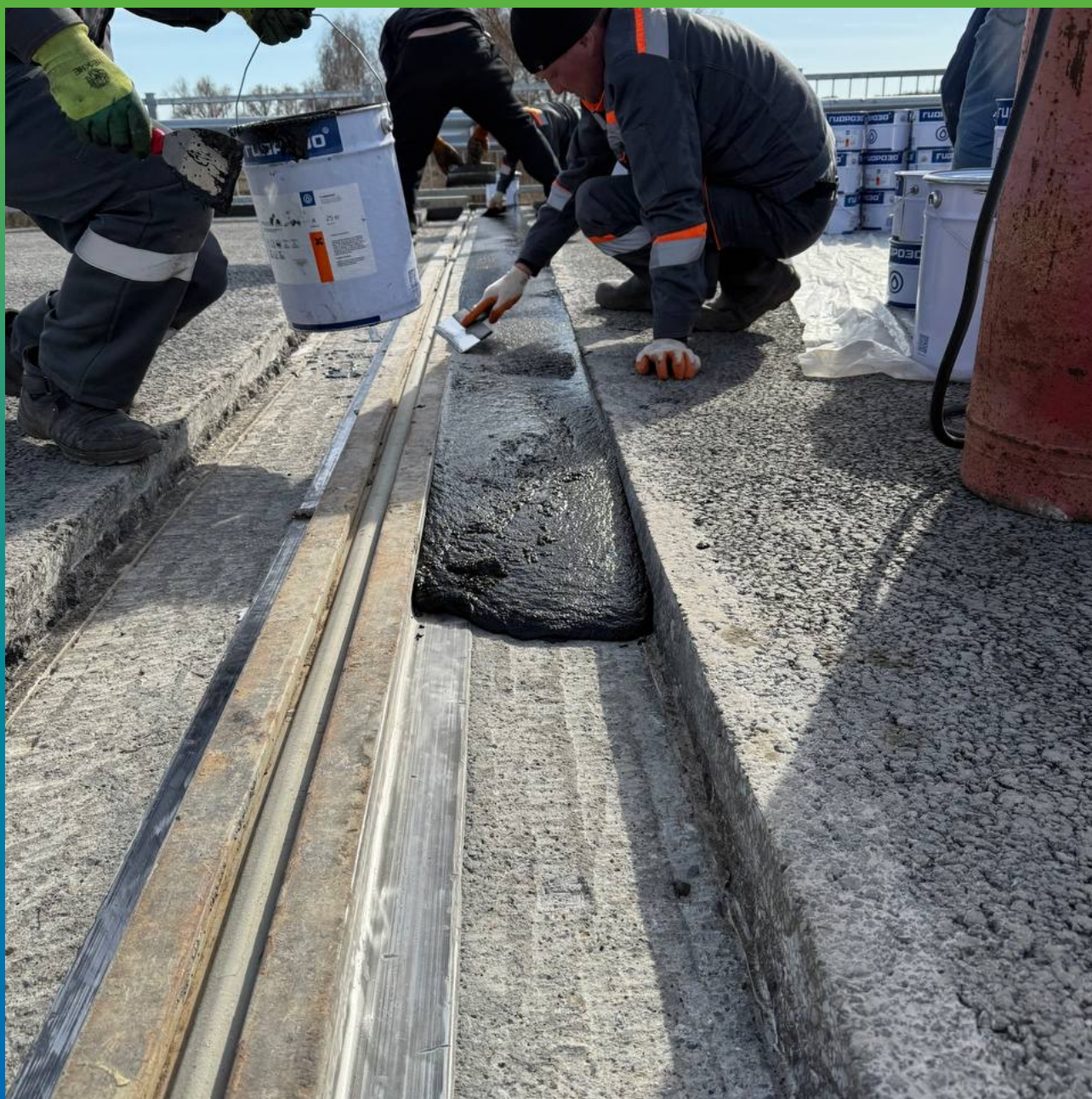
Распределение материала в штрабе
