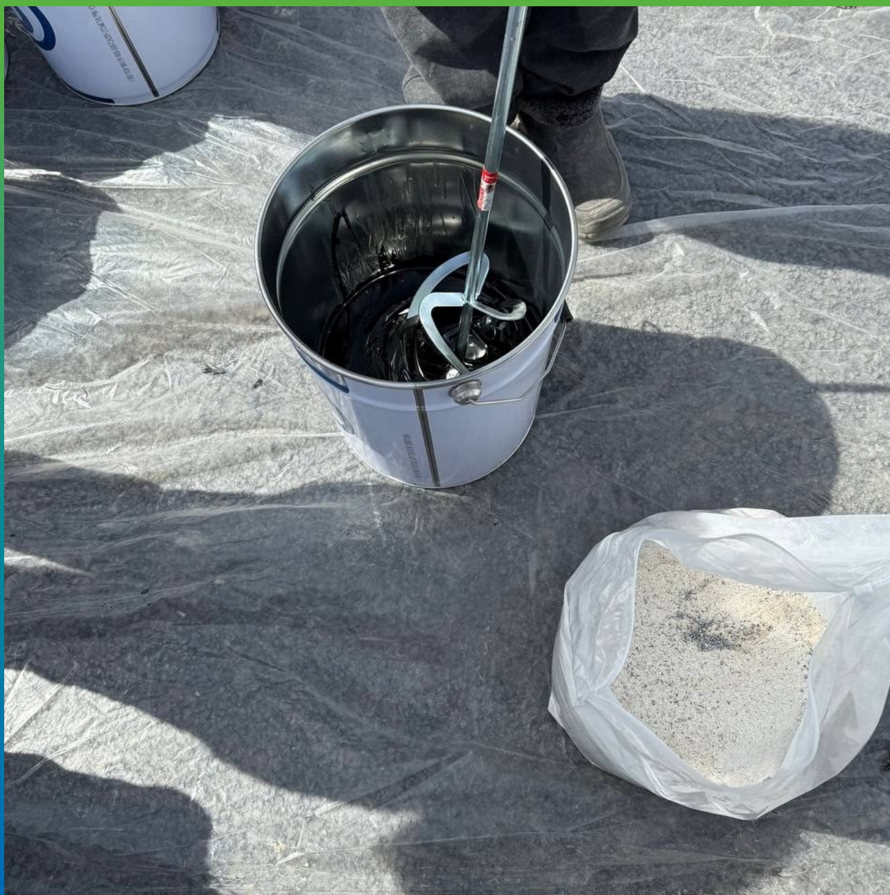
Смешивание компонентов Б1 и Б2 трехкомпонентного полиуретанового состава Манопур 336
