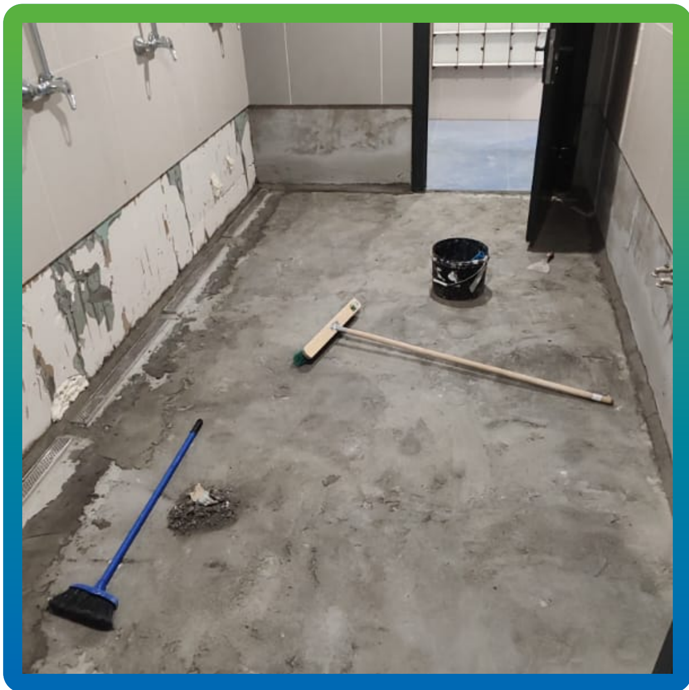
Ремонт основания и устройство галтелей материалом Стармекс РМЗ
