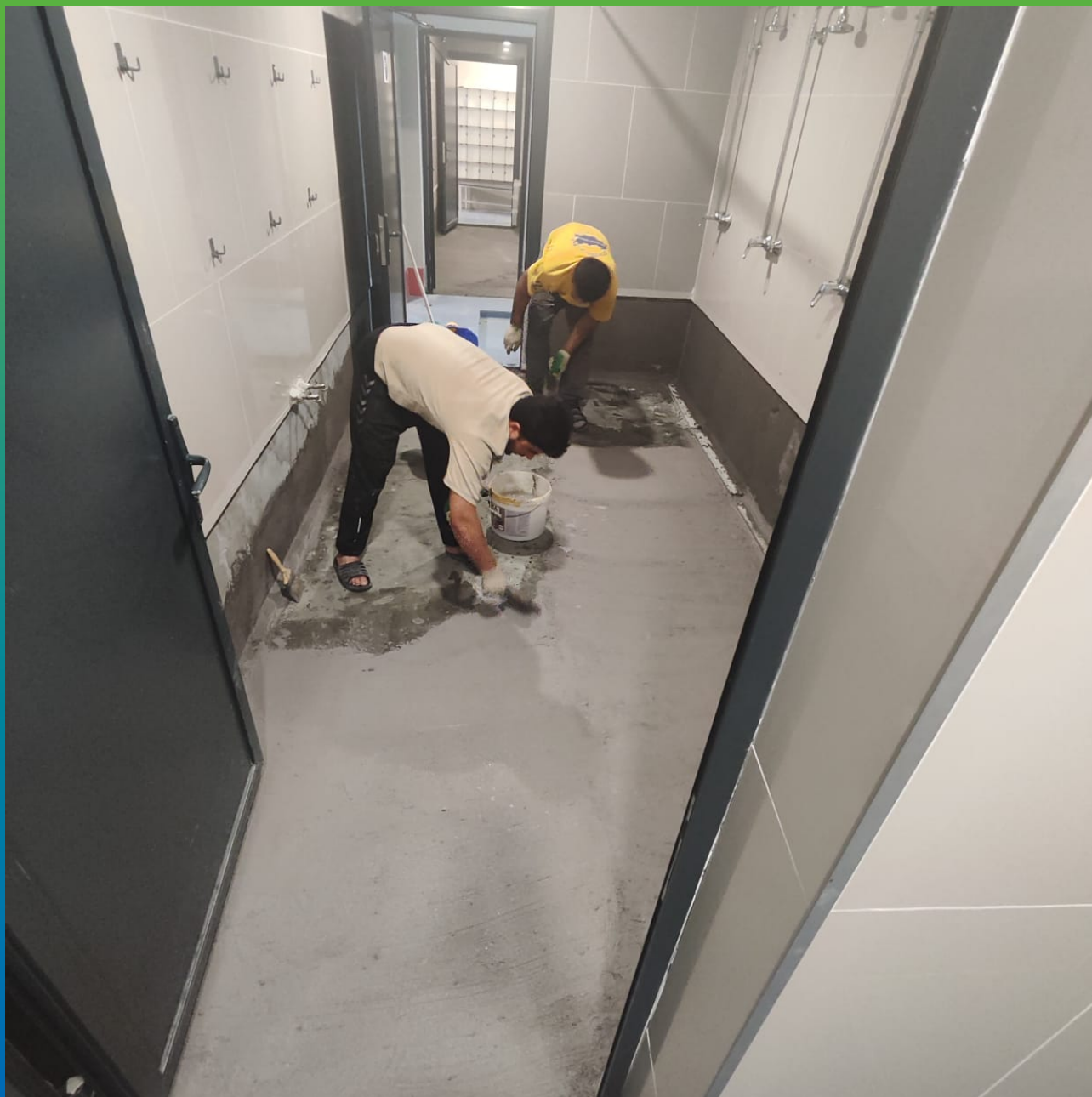
Нанесение эластичной полимерцементной гидроизоляции Стармекс Сил Флекс
