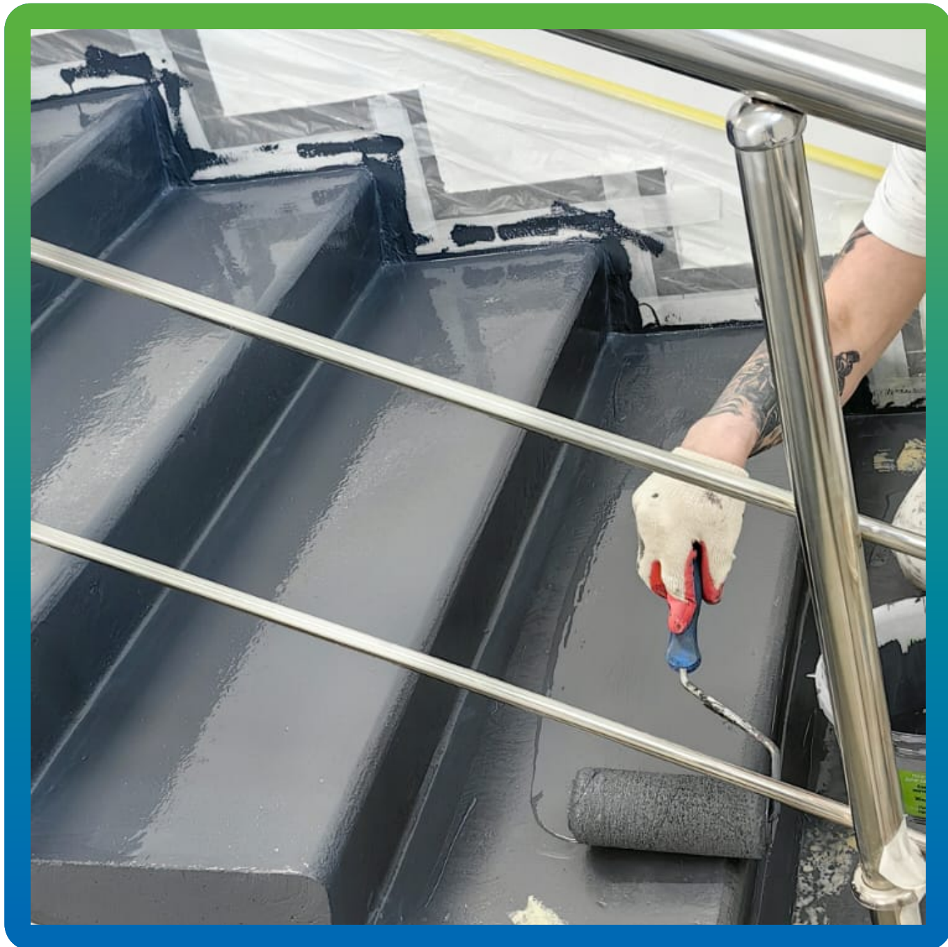
Нанесение ДенсТоп ПУ 302 (третий слой) + флокирование ДенсТоп Флокс СТ
