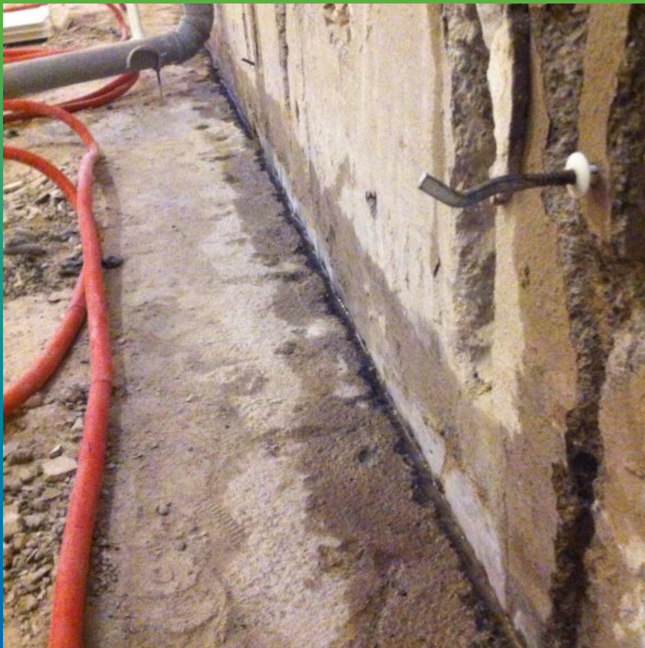
Расшивка стыка "стена-пол"
