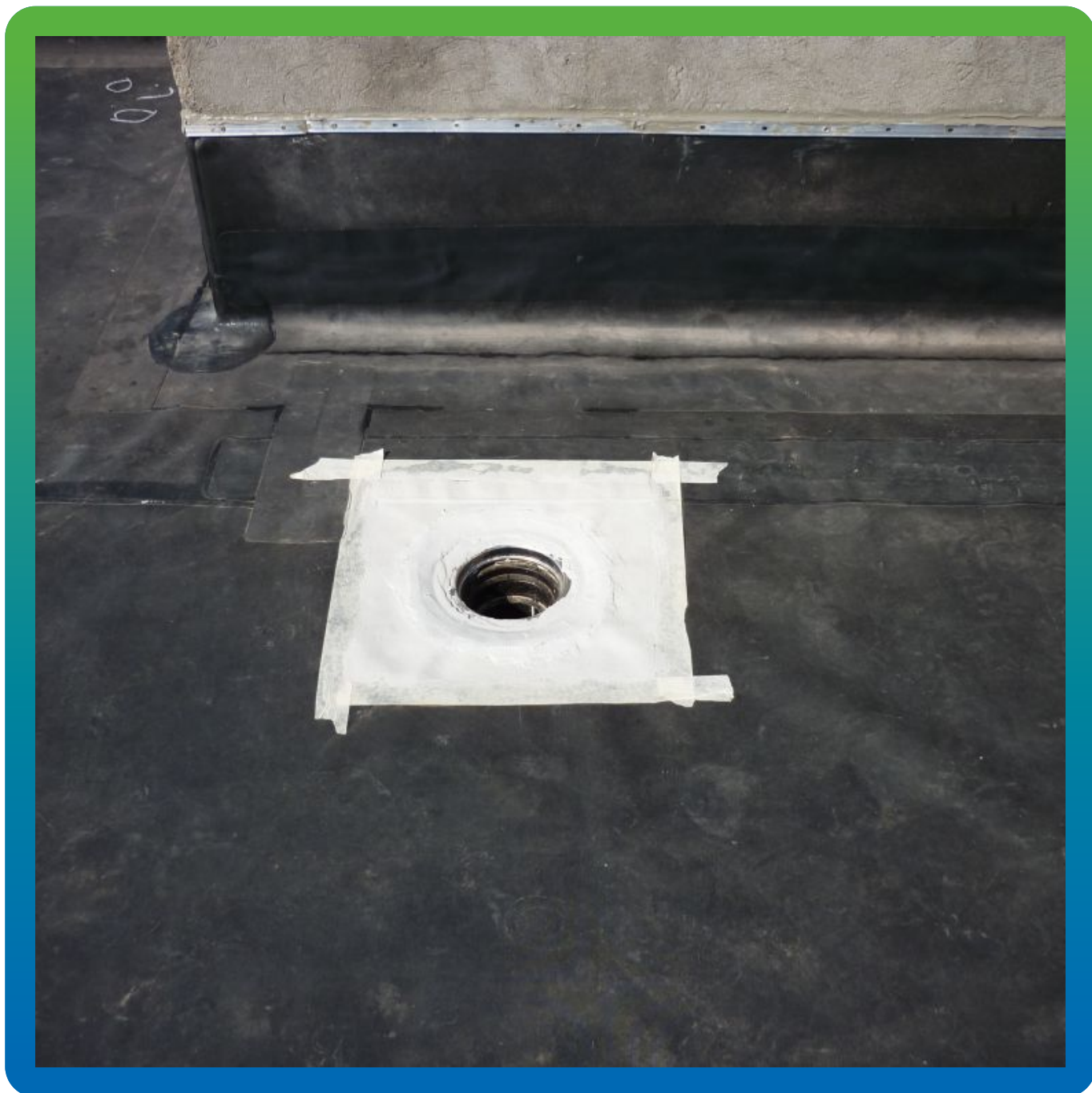
Устройство воронки с применением Максэластик Пур
