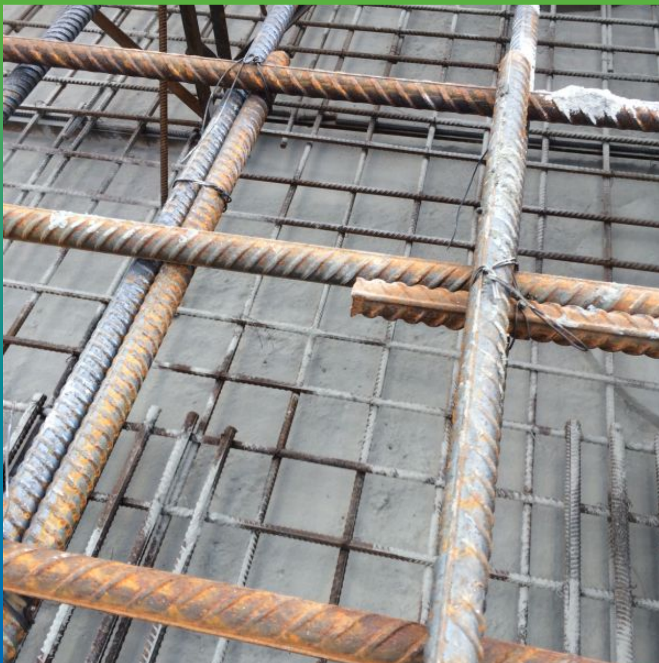
Просыпка Макссил Супер по нижнему поясу арматуры
