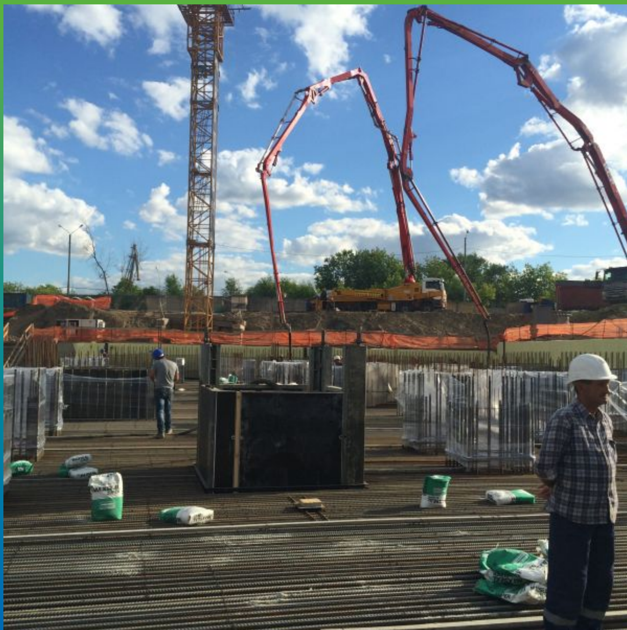
Подача бетона
