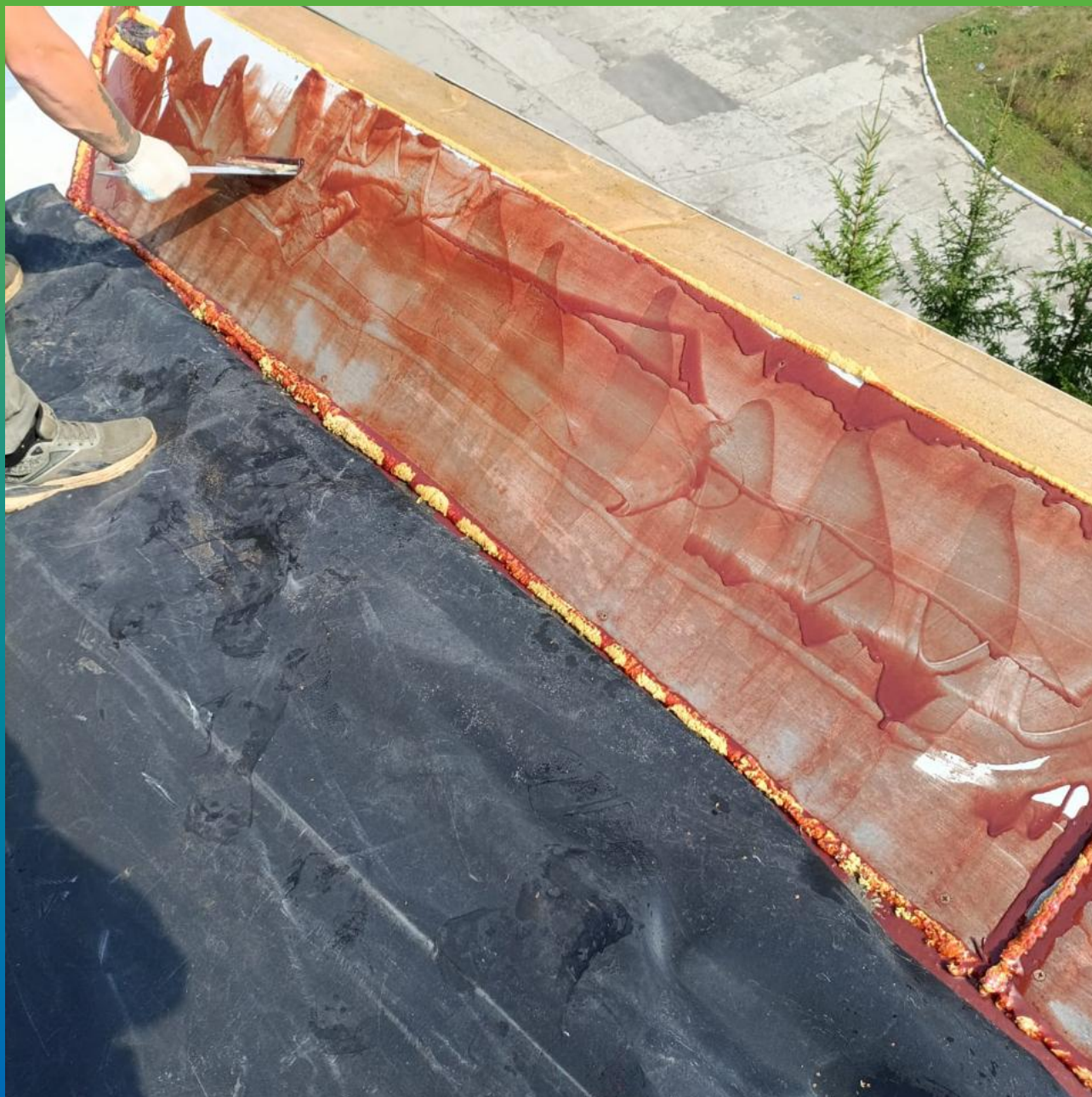
Нанесение материала Адгезив П400
