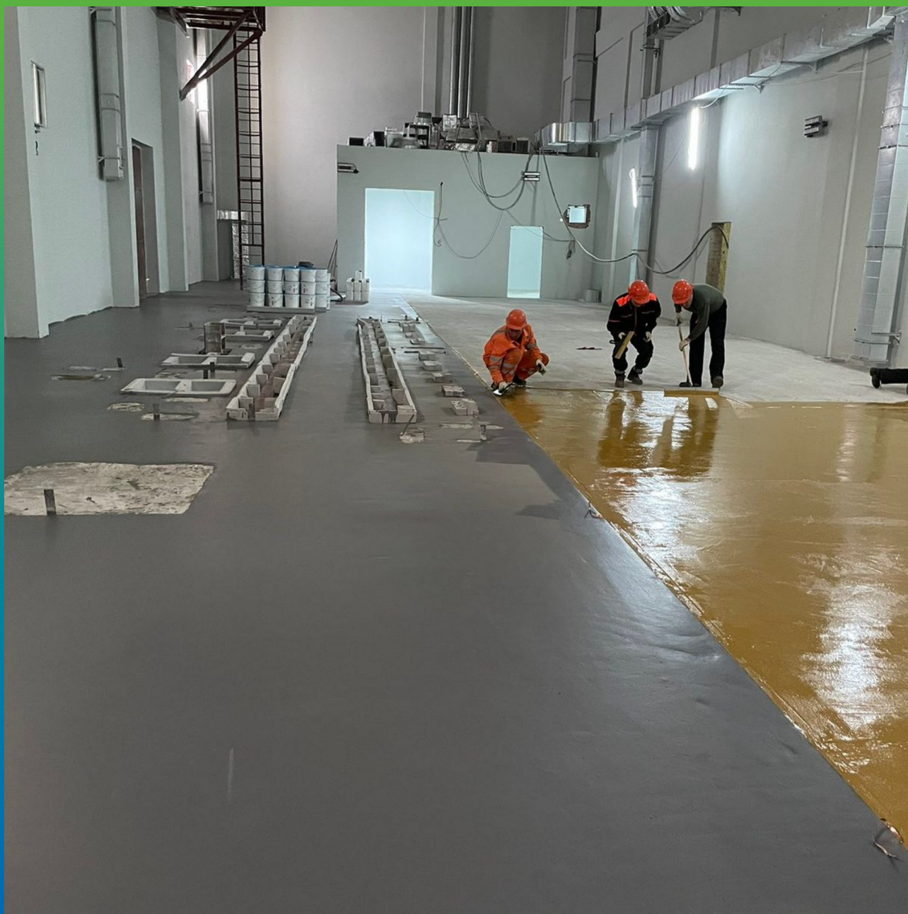
Грунтование основания материалом ДенсТоп ПМ 601, общий вид захватки
