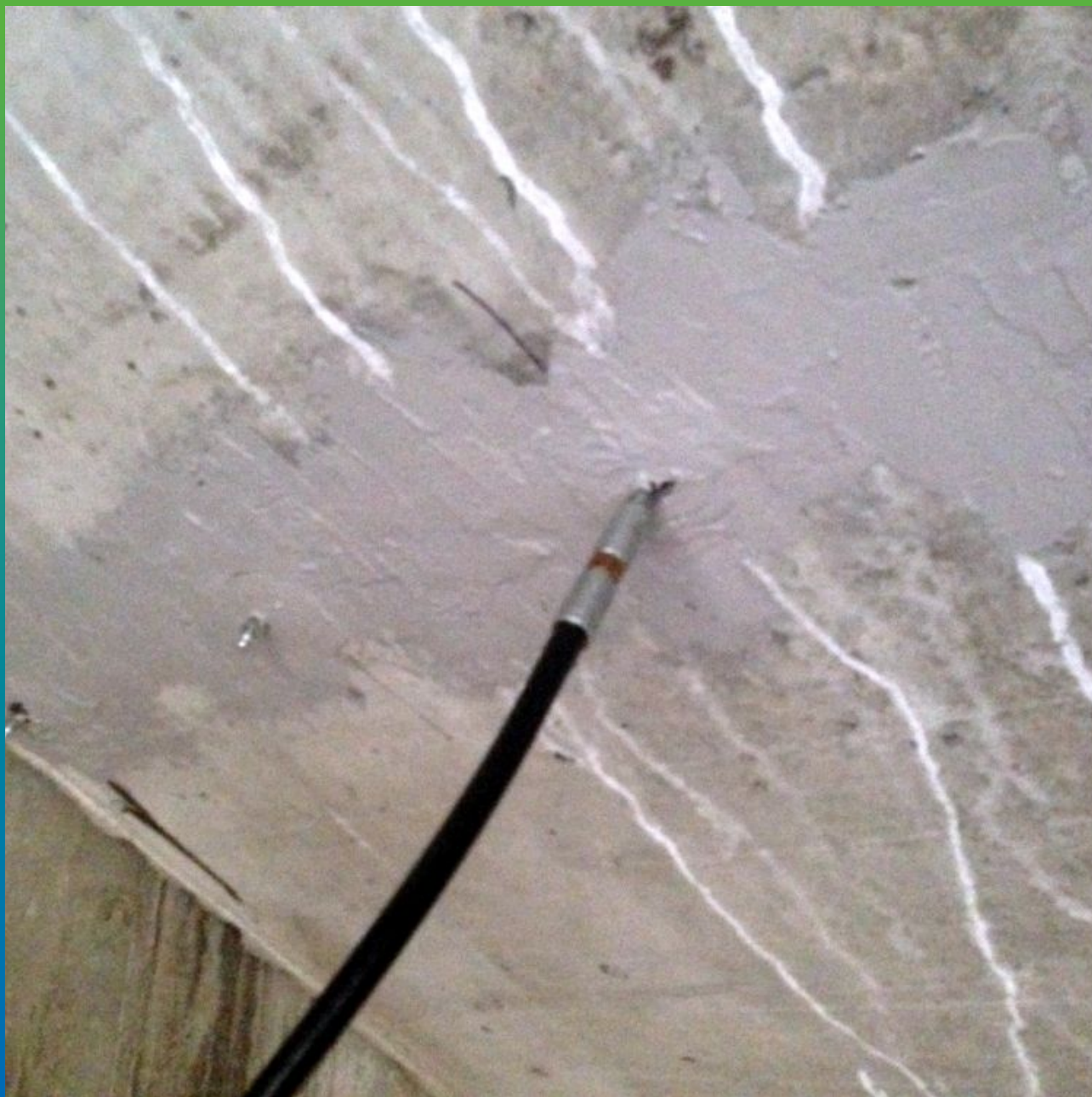
Последовательное заполнение пакеров на трещине. Общий вид.
