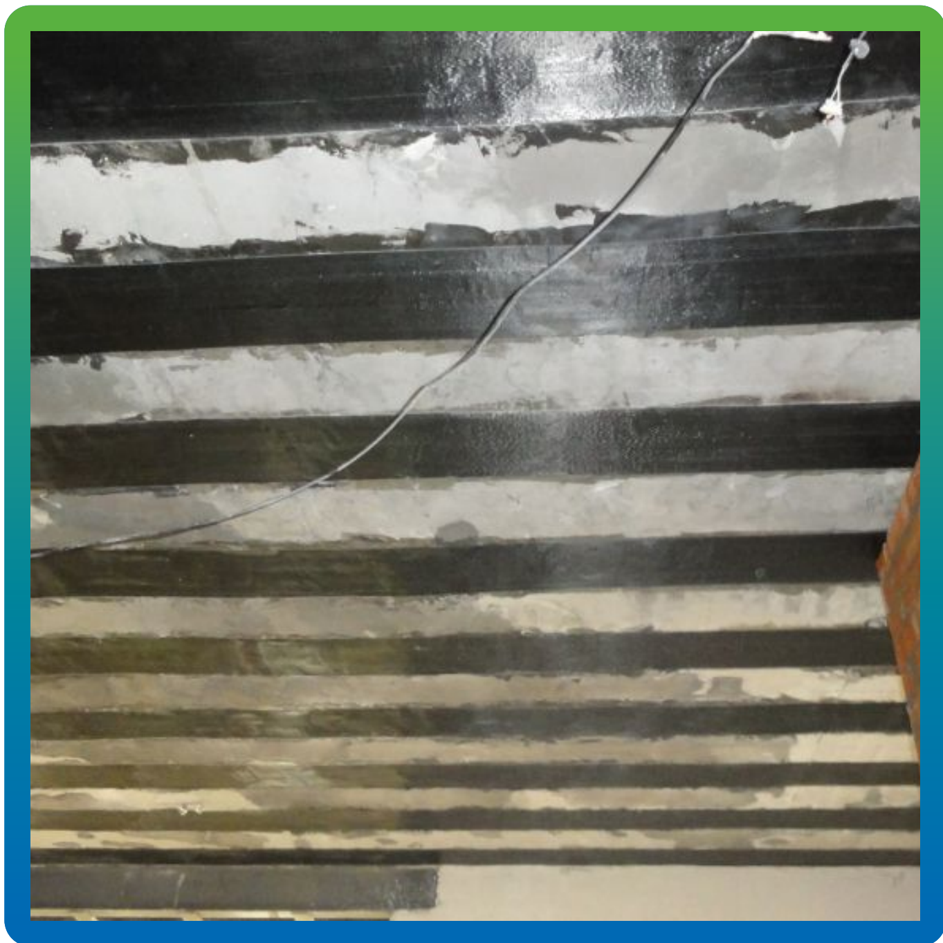
Финальный вид плиты перекрытия после окончания работ
