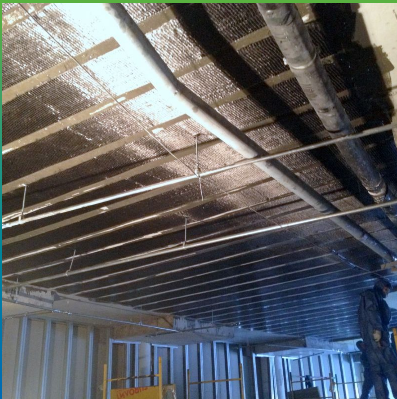
Общий вид смонтированной системы внешнего армирования углеродным волокном Армошел KB 900.
