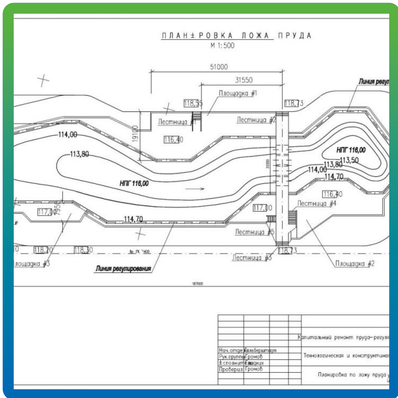
План водоема
