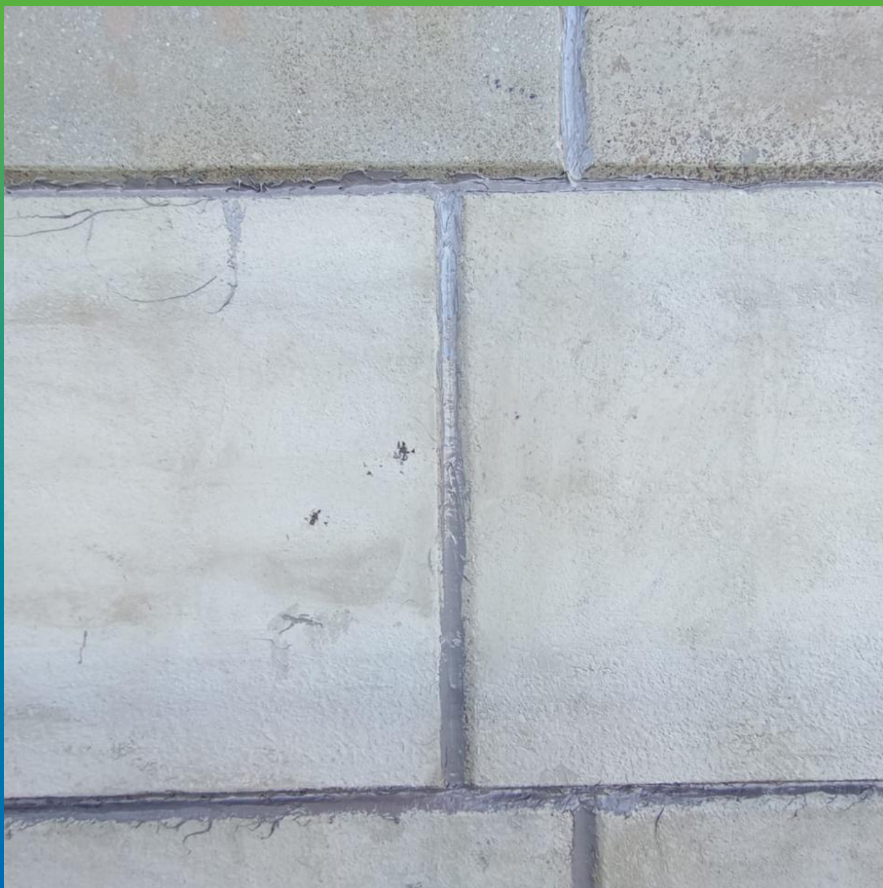
Герметизация швов кладки из железобетонных блоков составом Манодил ПС 190
