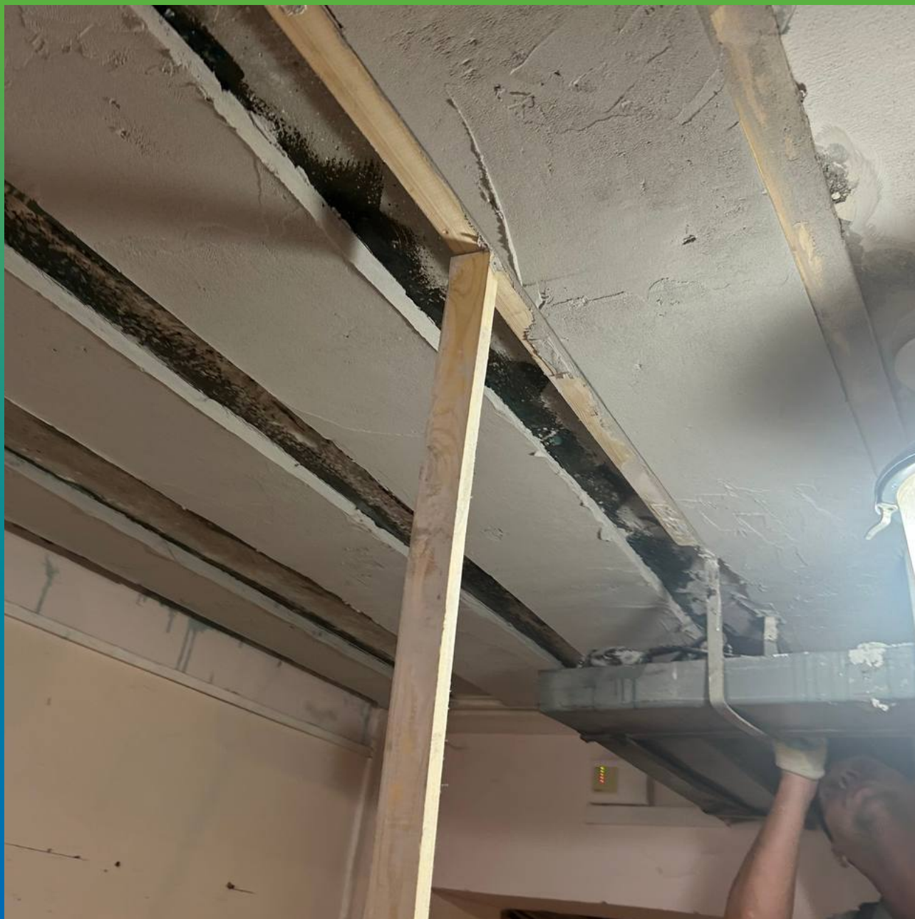
Монтаж огнезащиты Пирошел Цем толщиной 40 мм.
