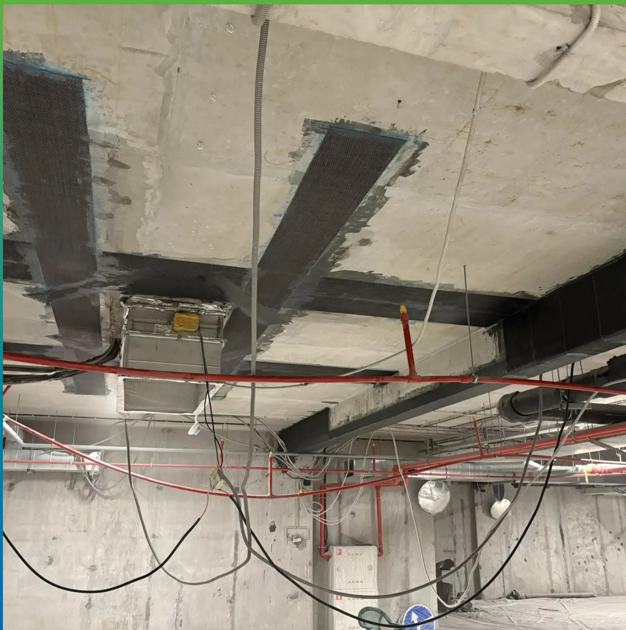
Монтаж углеволокна Армошел KB 900
