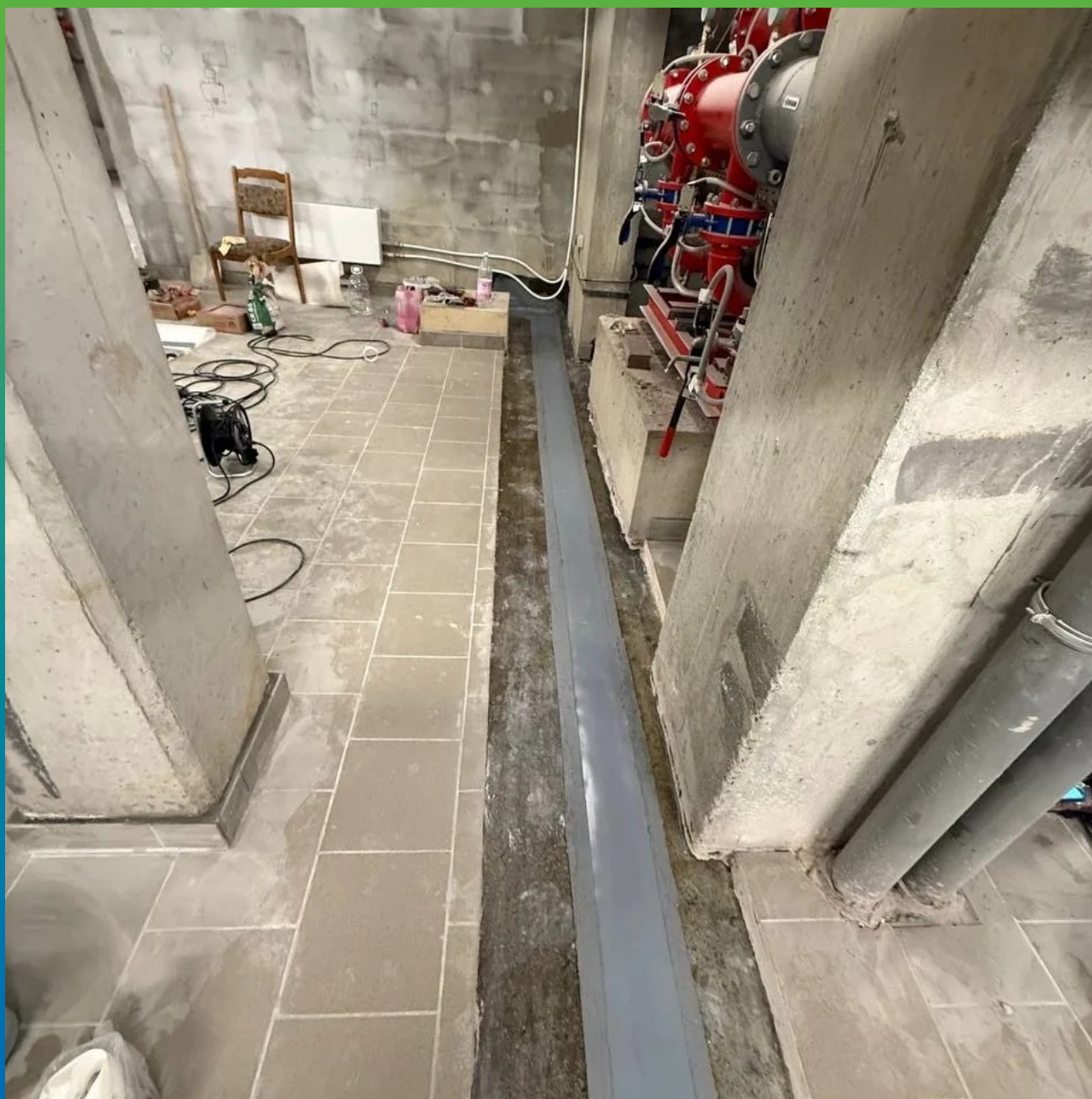
Вид смонтированной ленты Манодил Про на Манопокс 331
