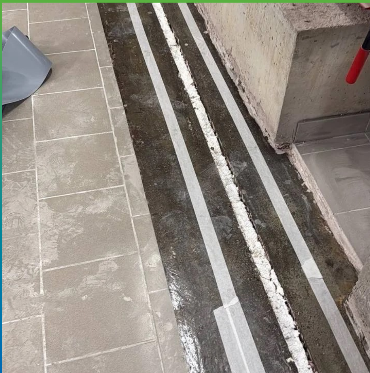
Приклейка малярного скотча перед монтажом ленты Манодил Про
