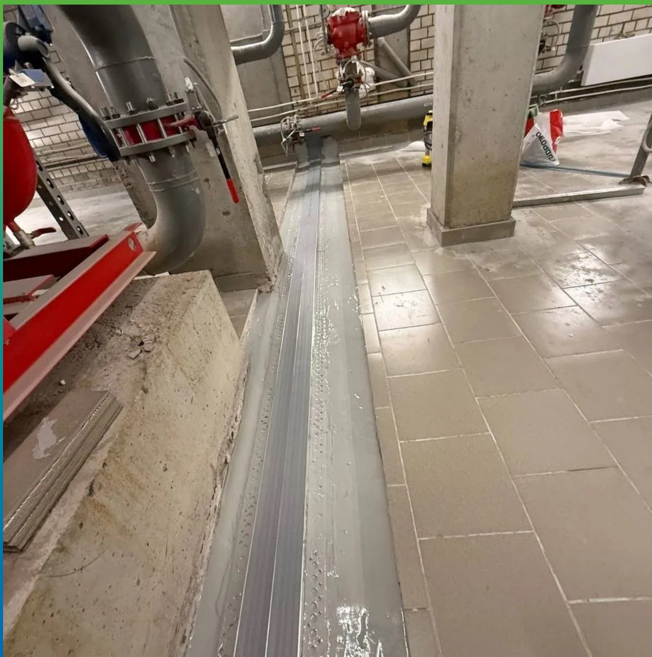
Вид нанесенного гидроизоляционного покрытия ДенТоп МС 351
