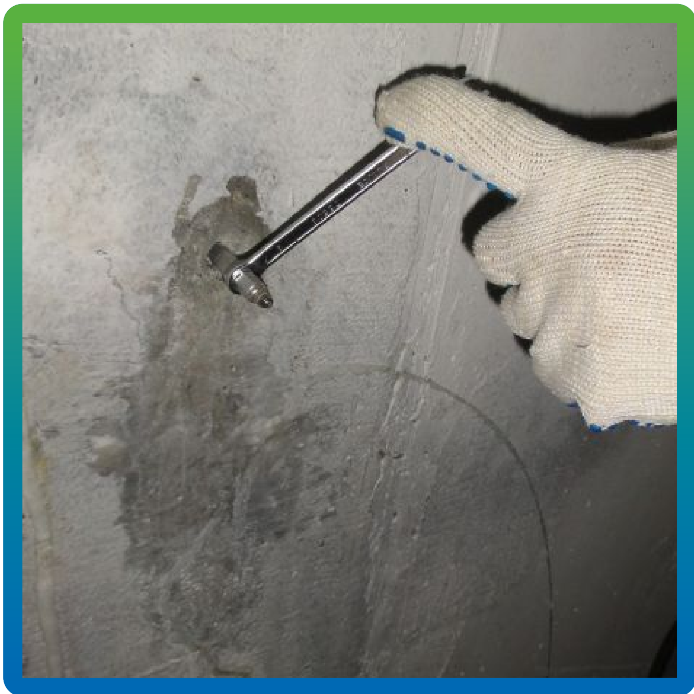
Установка инъекционных пакеров
