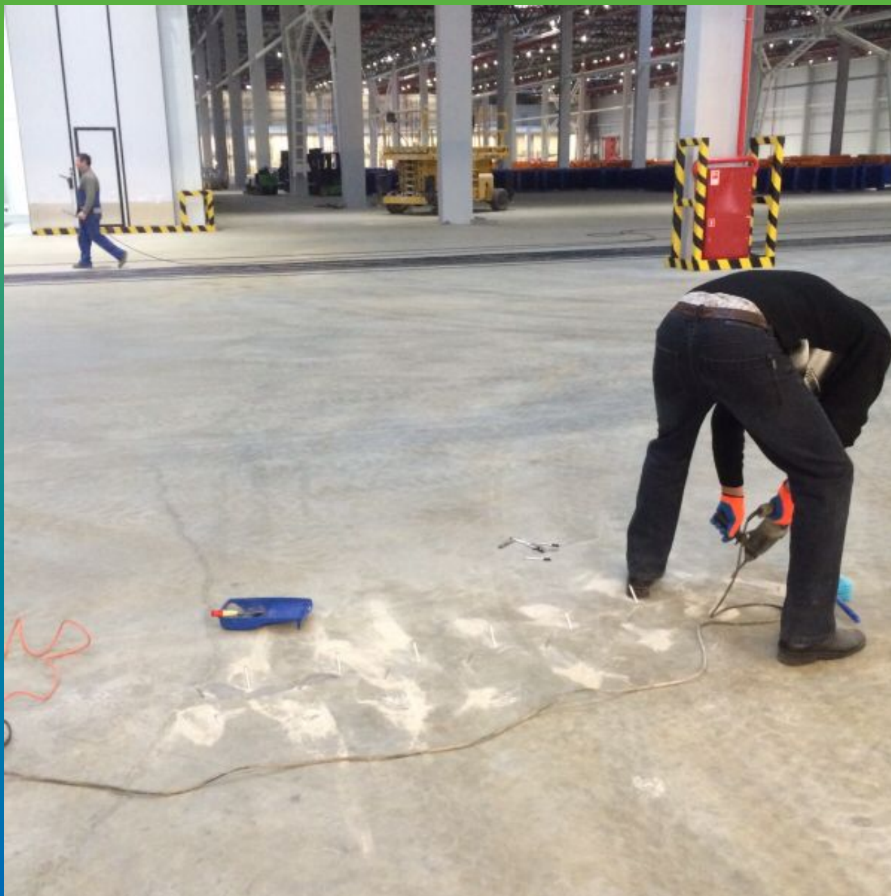
Сверление шпуров под пакеры БМ 1089
