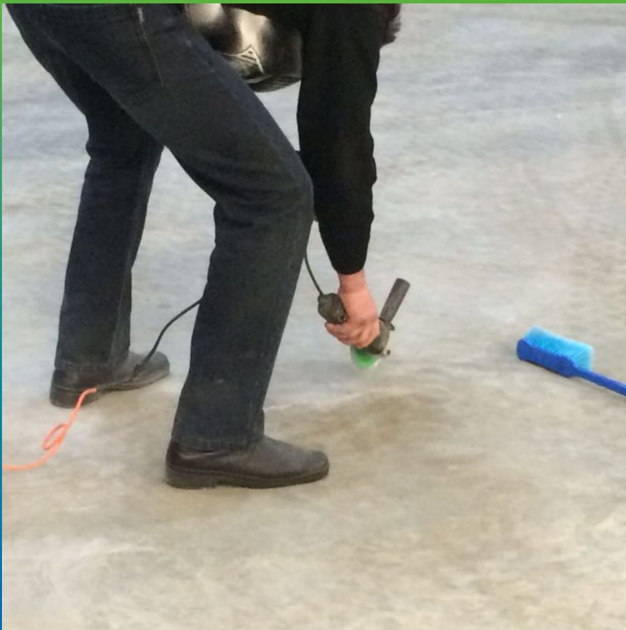
Подготовка трещин перед инъектированием Манопокс 352
