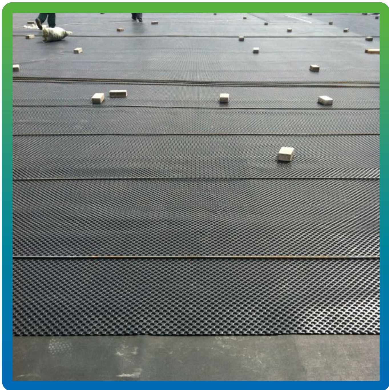
Устройство керамзитобетонного слоя с применением Максдрейн 8 ГТ
