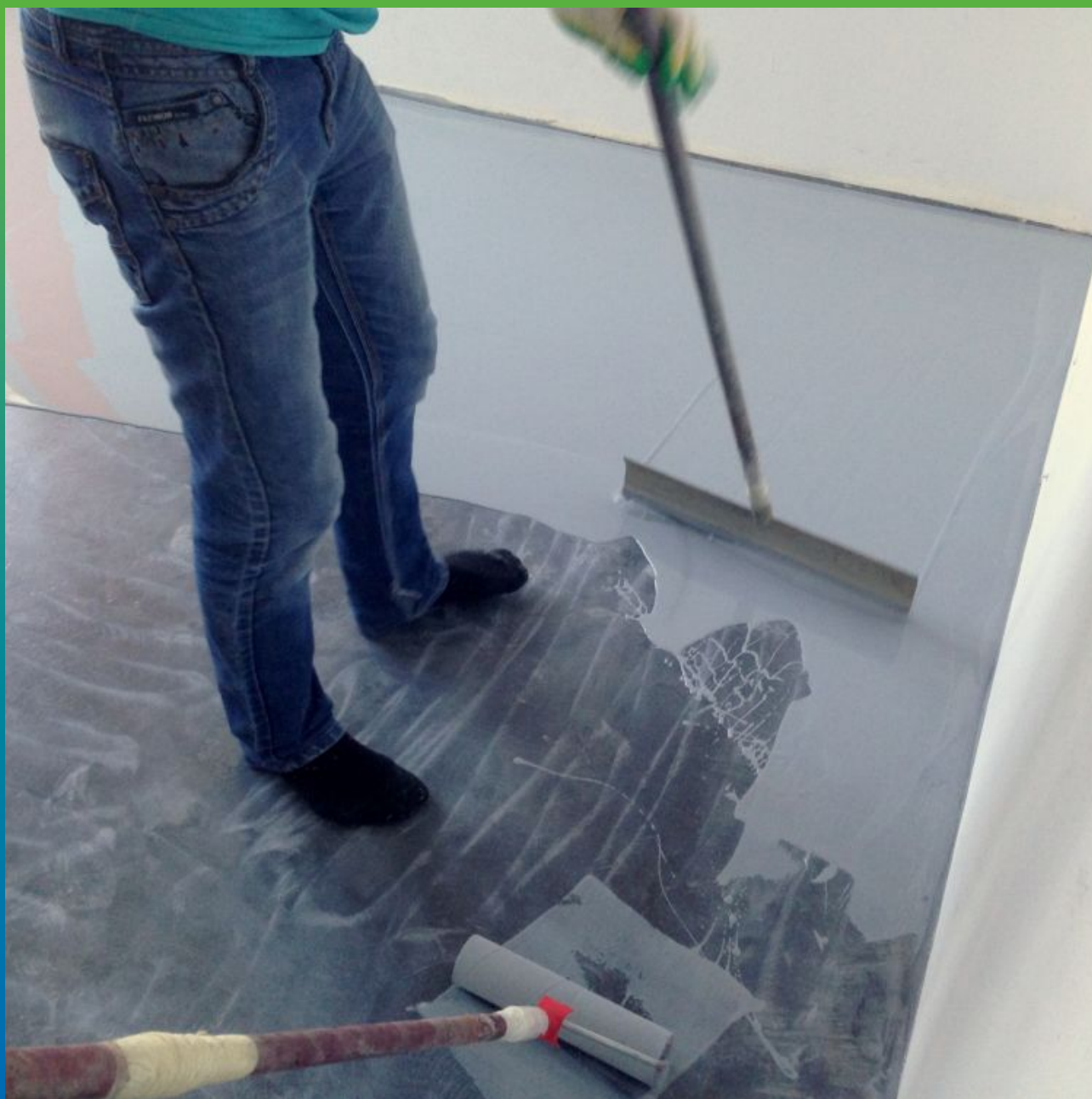
Распределения материала ракелью с регулируемой толщиной слоя.
