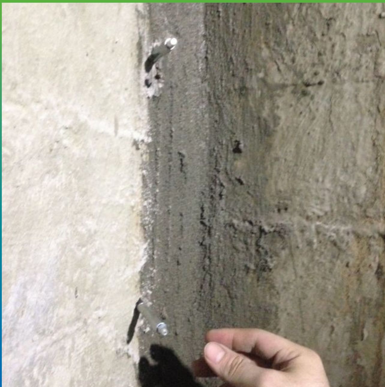
Установка пакеров БМ 1133.
