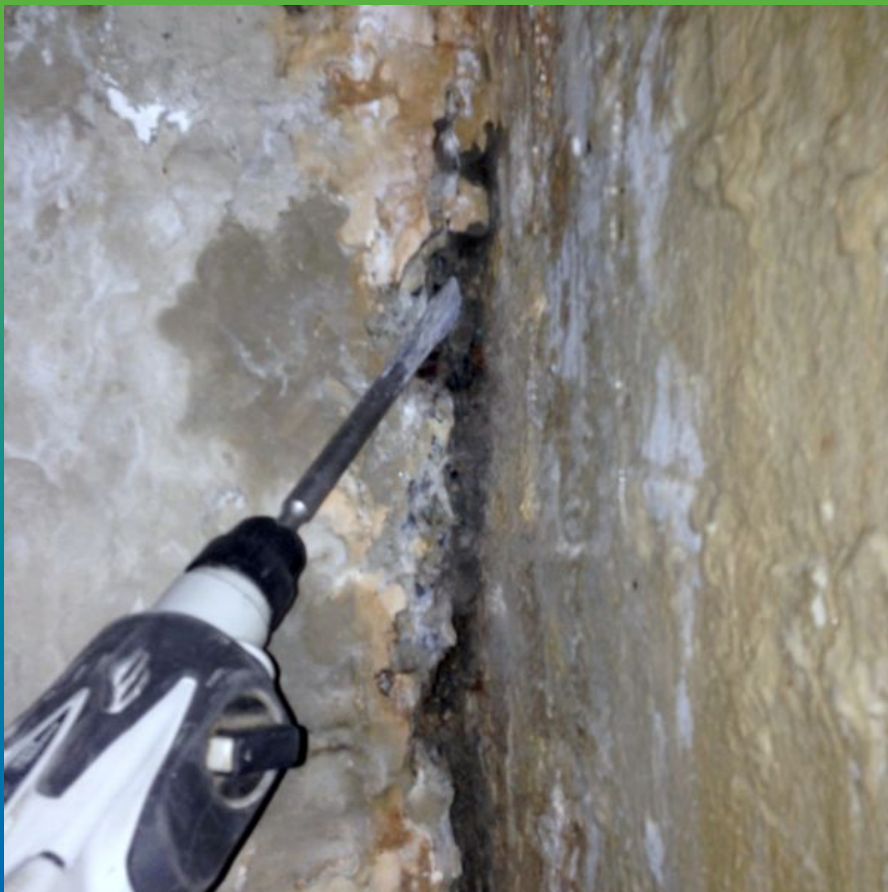
Штрабление. Удаление ремонтного состава.
