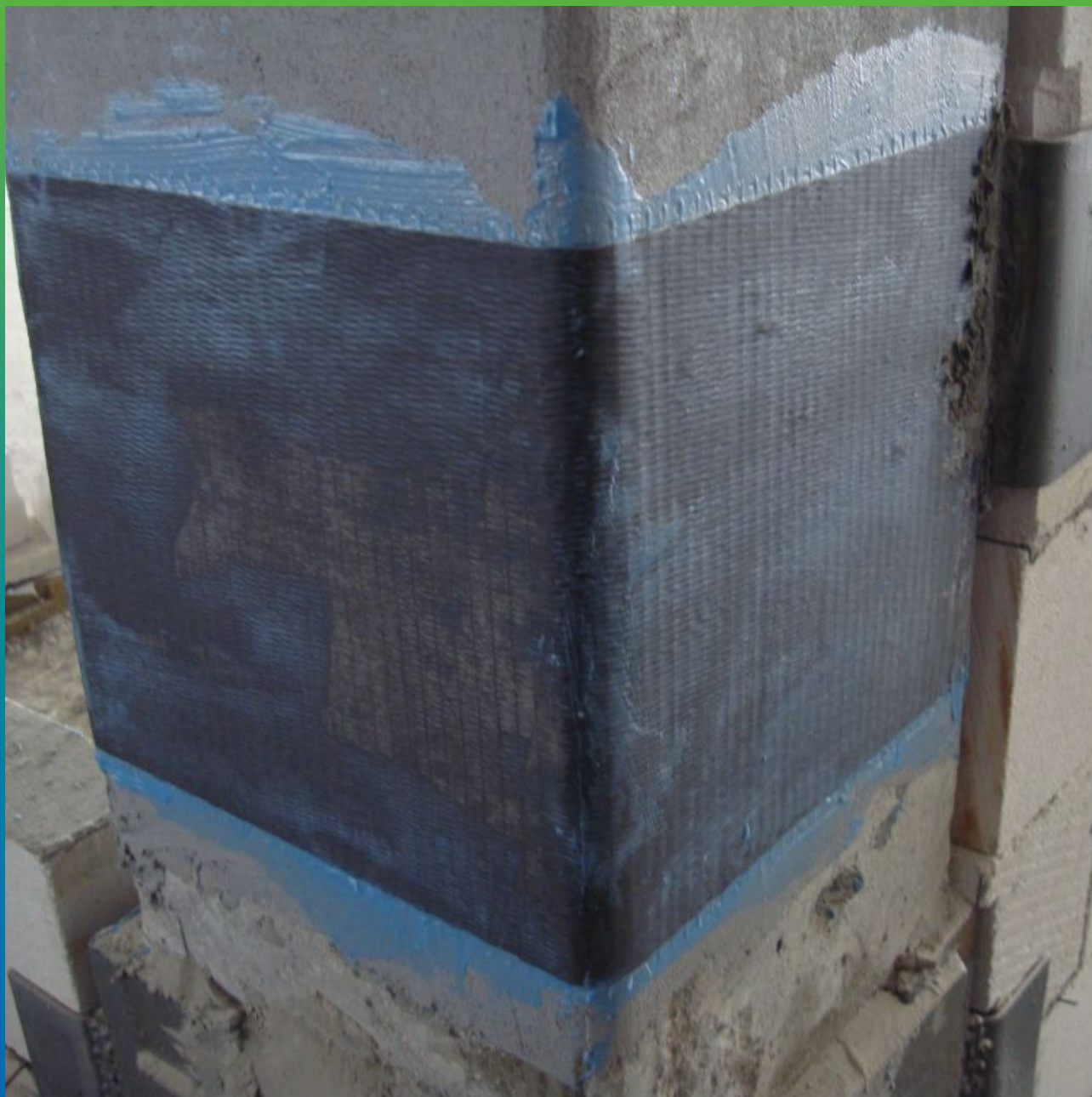
Усиление колонны с применением Манопокс 183
