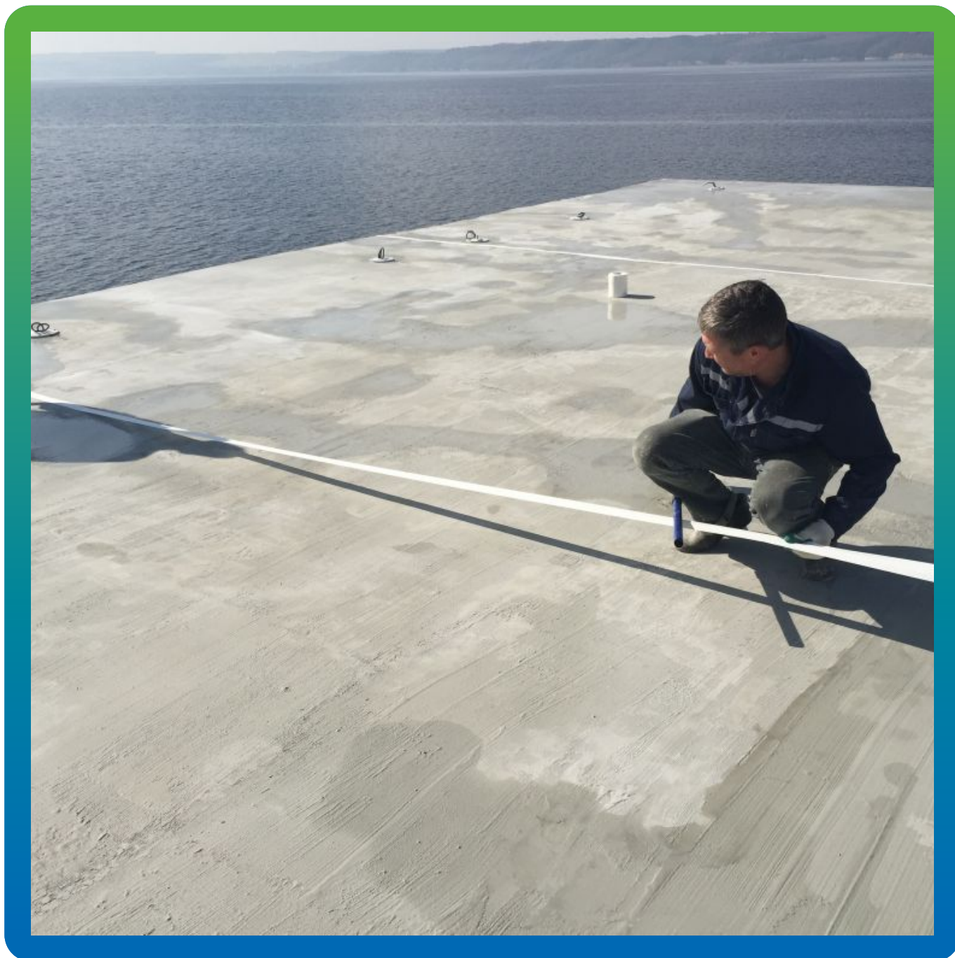
Разметка поверхности перед нанесением третьего слоя Макссил Флекс
