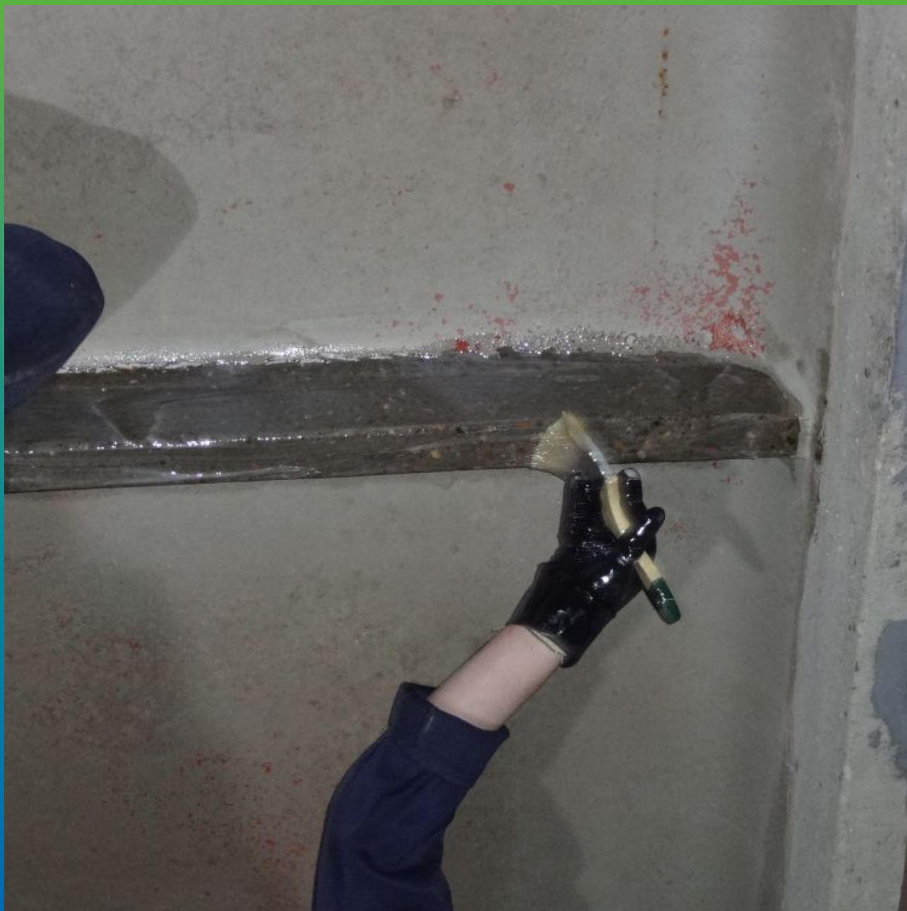
Нанесение на поверхность загущённого эпоксидного состава Манопокс 372
