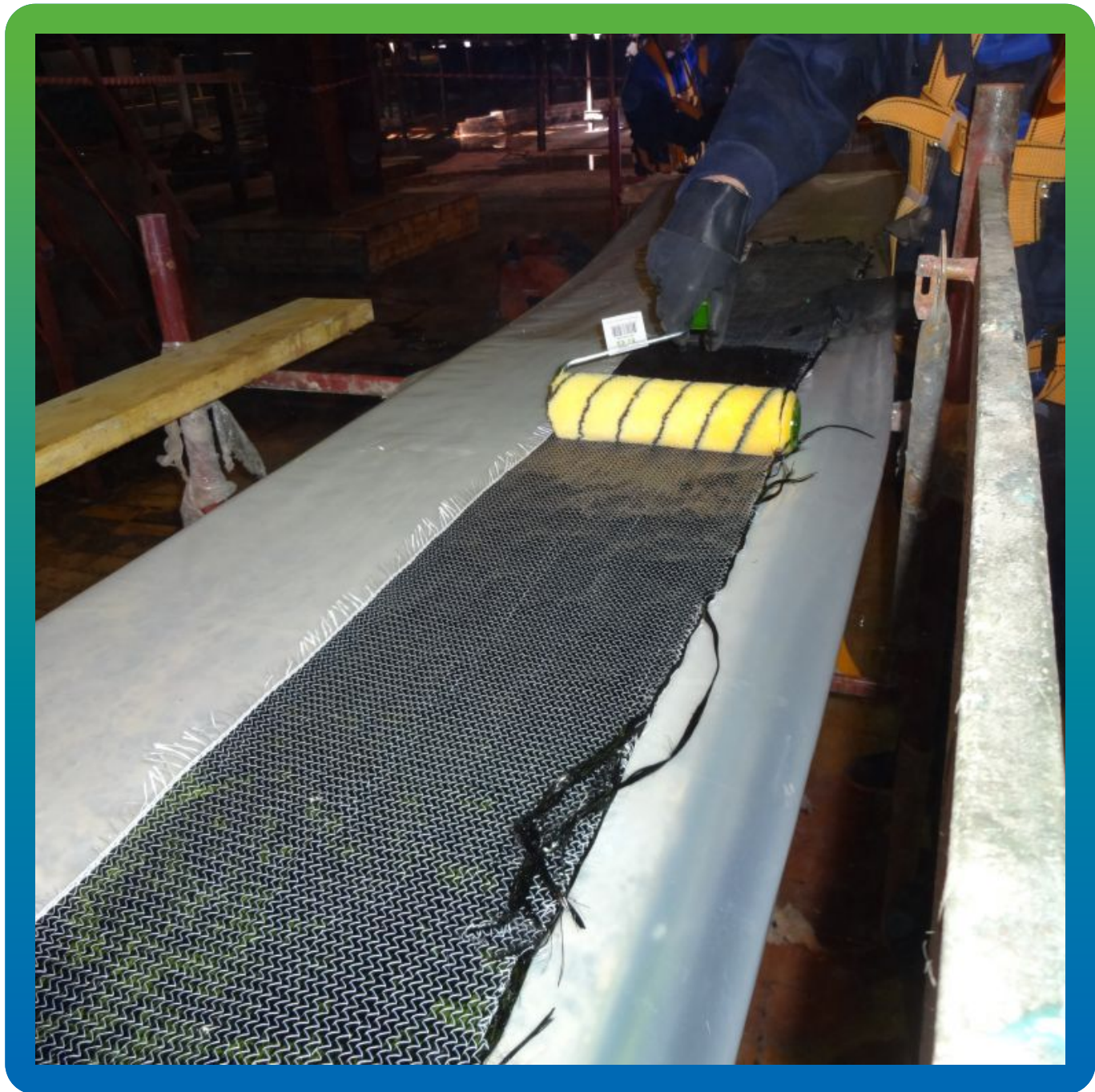
Пропитка углеродного холста эпоксидным составом Манопокс 372
